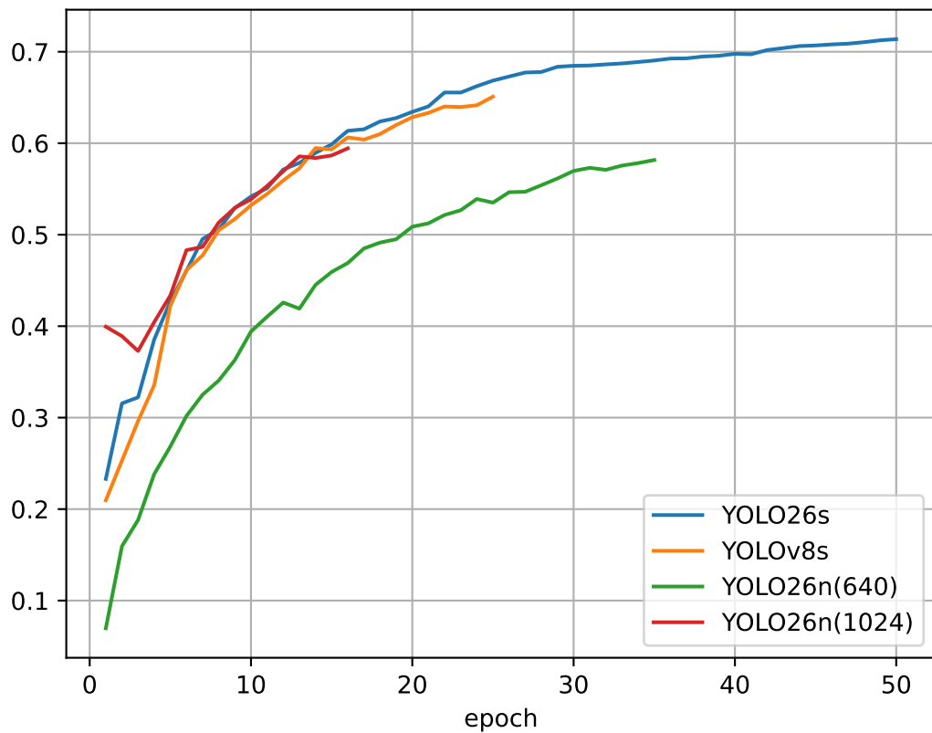
mAP50-95(B)
