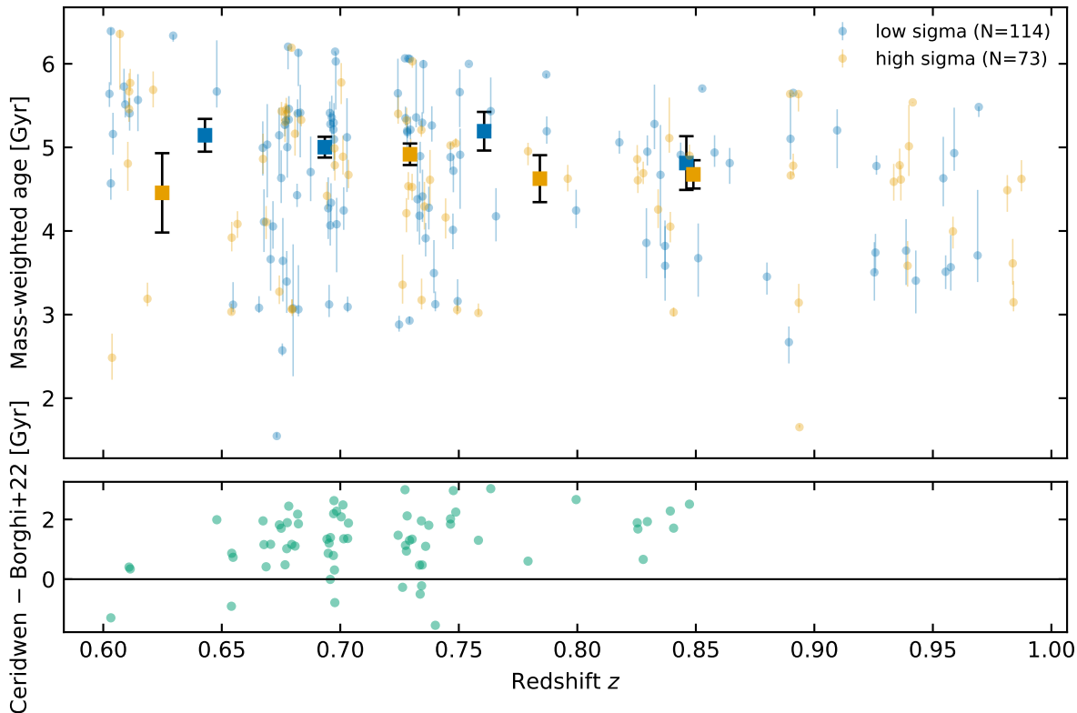
Ceridwen DR2 quiescent ages vs redshift (N=187)
