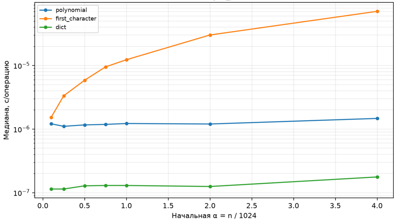
ЛП 8: get_hit
