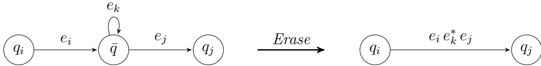
Figure 12: Eliminazione dello stato \bar{q} : il cammino q_i \rightarrow \bar{q} \rightarrow q_j con cappio su \bar{q} diventa un'unica transizione etichettata da e_i e_k^* e_j .
