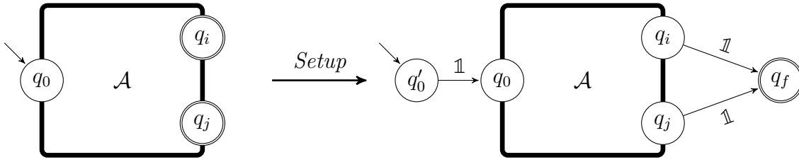
Figure 9: Trasformazione dell'automa \mathcal{A} dopo Setup.
