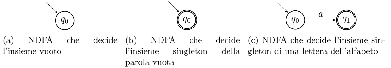
Figure 6: Gli automi che decidono le tre espressioni regolari di base
