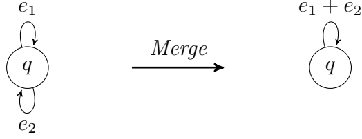
Figure 11: Caso particolare del Merge con q_i = q_j = q : due cappi su q sono transizioni parallele da q a q , e vengono fusi in un unico cappio etichettato da e_1 + e_2 .
