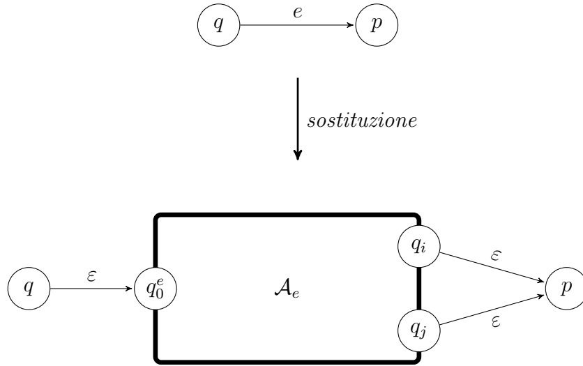
Figure 8: Un passo di sostituzione: la transizione T(q, e) = p viene rimpiazzata dal DFA \mathcal{A}_e che decide \llbracket e \rrbracket , collegato a q e a p tramite \epsilon -transizioni.
