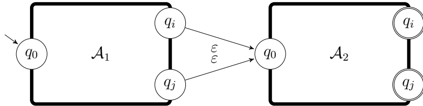
Figure 4: L'idea della dimostrazione consiste nel costruire un automa usando le \epsilon -mosse per concatenare le computazioni dei due automi.
