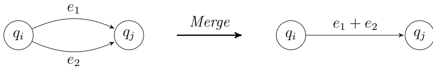
Figure 10: Fusione di due transizioni parallele da q_i a q_j in un'unica transizione etichettata dalla somma delle espressioni regolari.
