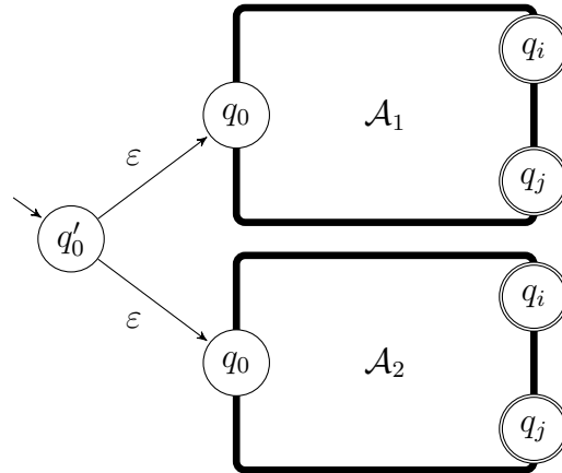
Figure 7: Costruzione dell'automa che decide X_1 + X_2 a partire da quelli che decidono X_1 e X_2 .
