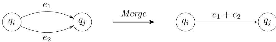
Figura 10: Fusione di due transizioni parallele da q_i a q_j in un'unica transizione etichettata dalla somma delle espressioni regolari.
