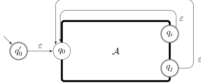
Figura 5: Costruzione dell'automa che decide X^* a partire da quello che decide X .
