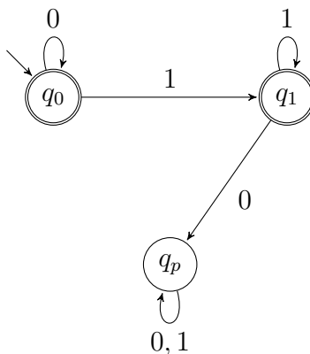
Figura 25: DFA che decide il linguaggio \{0^n 1^m \mid n, m \in \mathbb{N}\} .
