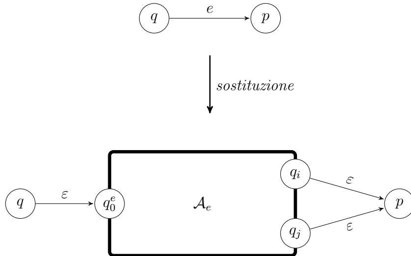
Figura 8: Un passo di sostituzione: la transizione T(q, e) = p viene rimpiazzata dal DFA \mathcal{A}_e che decide \llbracket e \rrbracket , collegato a q e a p tramite \epsilon -transizioni.
