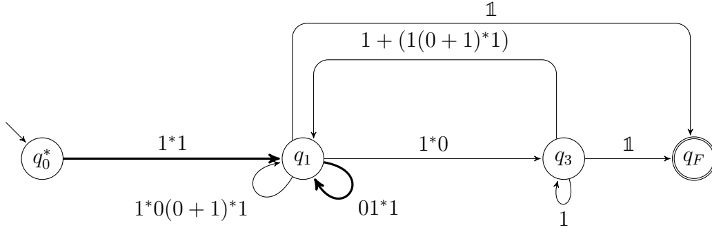
Figura 20: Passo 6, eliminazione di q_0 .
