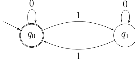
Figura 2: In modo simile all'automa dell'Esempio 2.6 si può dare l'automa che decide l'insieme di tutte le parole con un numero pari di 1.
