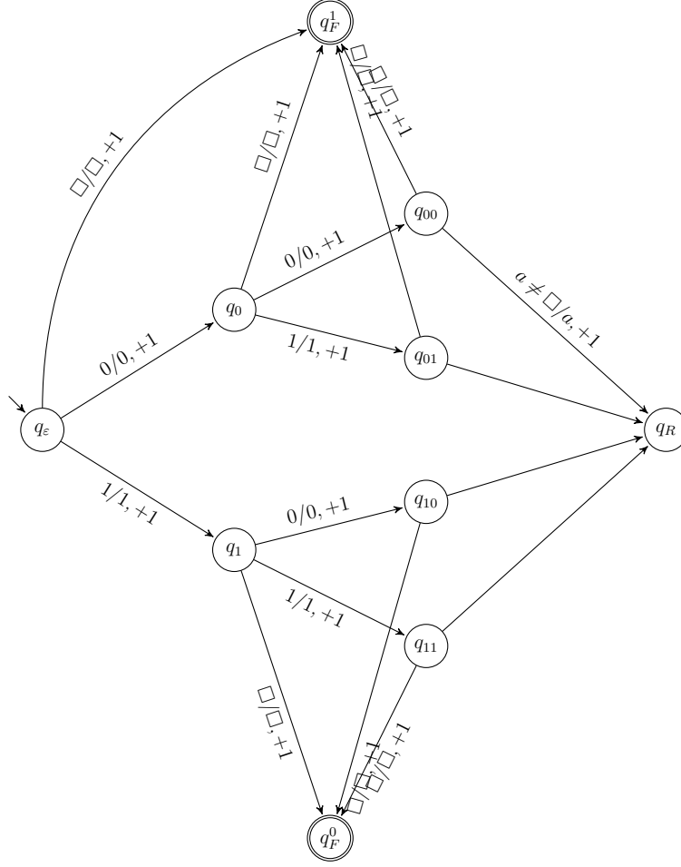
Figura 28: Stati q_w di \mu' per A = \{0, 1\} , N = 2 e X \cap A^{\leq 2} = \{\epsilon, 0, 00, 01\} : le parole in X portano in q_F^1 , le altre in q_F^0 .
