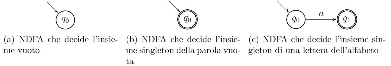
Figura 6: Gli automi che decidono le tre espressioni regolari di base
