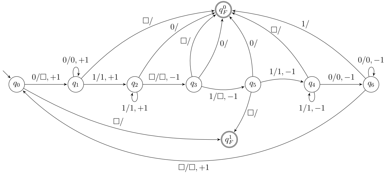
Figure 26: Macchina di Turing che decide X = \{0^n 1^n \mid n \in \mathbb{N}\} : accetta in q_F^1 e rifiuta in q_F^0 .
