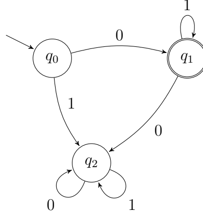
Figura 3: Automata che decide l'insieme X = \{01^n \mid n \geq 0\} .
