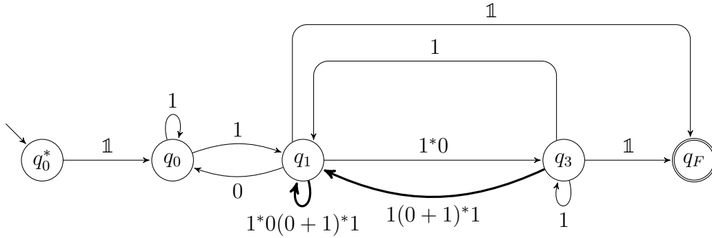
Figura 18: Passo 4, eliminazione di q_6 .
