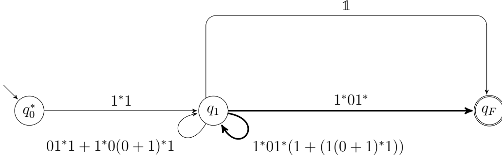
Figura 22: Passo 8, eliminazione di q_3 .
