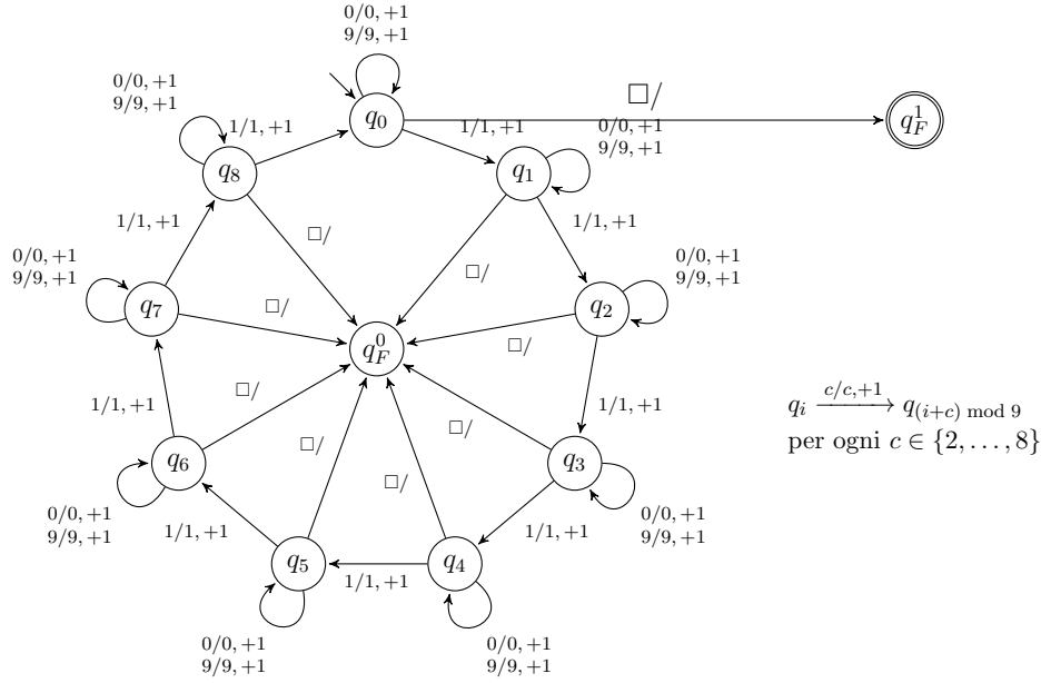
Figure 27: Macchina di Turing che decide la divisibilità per 9. Gli stati q_0, \dots, q_8 memorizzano il resto modulo 9 della somma delle cifre lette finora, con q_0 stato iniziale. Leggendo una cifra c in q_i , la macchina la riscrive invariata, si sposta a destra e passa in q_{(i+c) \bmod 9} : i cappi corrispondono alle cifre 0 e 9, gli archi tra stati consecutivi alla cifra 1, mentre le cifre 2, \dots , 8 sono riassunte nella legenda. Alla lettura del simbolo vuoto \square , la macchina accetta in q_F^1 se si trova in q_0 (resto 0) e rifiuta in q_F^0 se si trova in uno degli stati q_1, \dots, q_8 .
