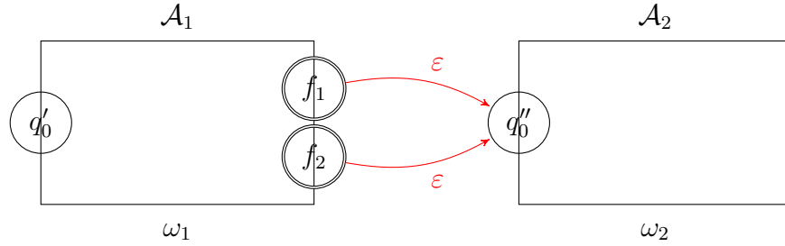
Figure 4: L'idea della dimostrazione per comporre in serie due automi e/' la seguente: usiamo le \epsilon -mosse per concatenare le computazioni dei due automi du due parole arbitrarie \omega_1, \omega_2 \in A^* (nella figura abbiamo F' = \{f_1, f_2\} ).
