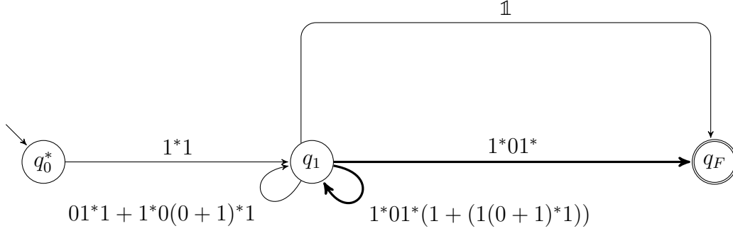
Figure 22: Passo 8, eliminazione di q_3 .
