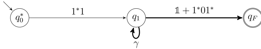
Figure 23: Passo 9, fusione dei cappi su q_1 e degli archi da q_1 a q_F .
