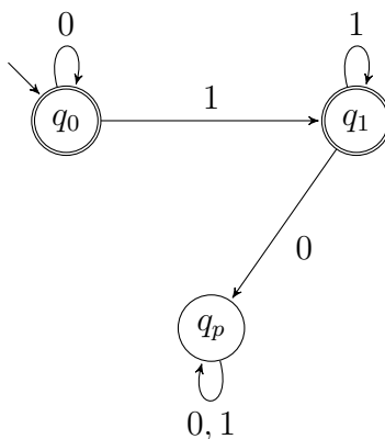
Figure 25: DFA che decide il linguaggio \{0^n 1^m \mid n, m \in \mathbb{N}\} .
