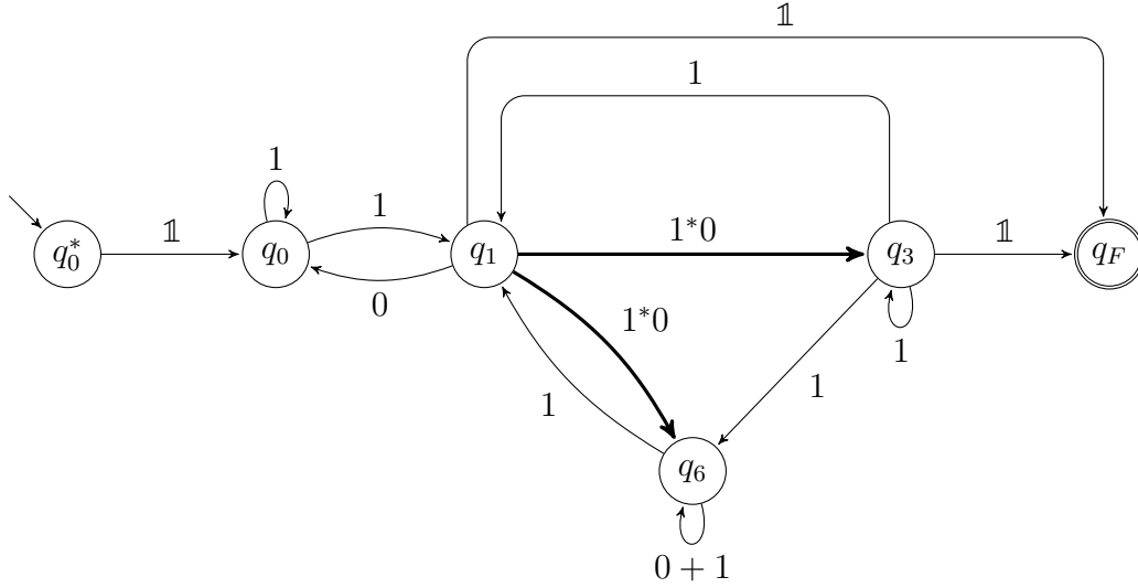
Figure 17: Passo 3, eliminazione di q_2 .
