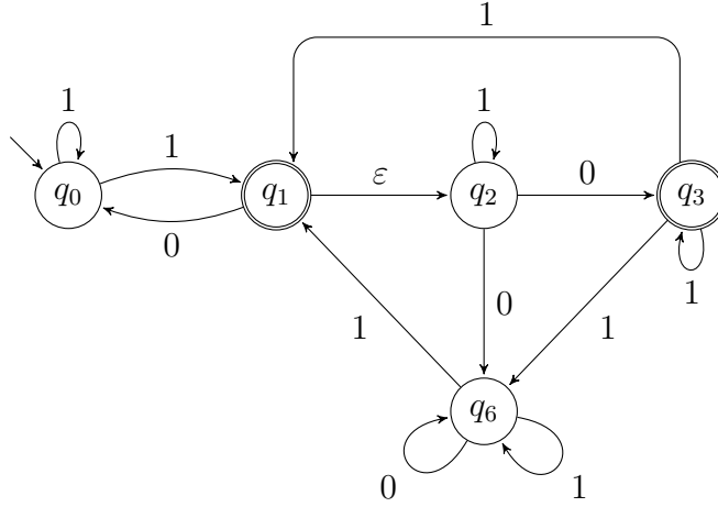
Figure 13: L'automata di partenza.
