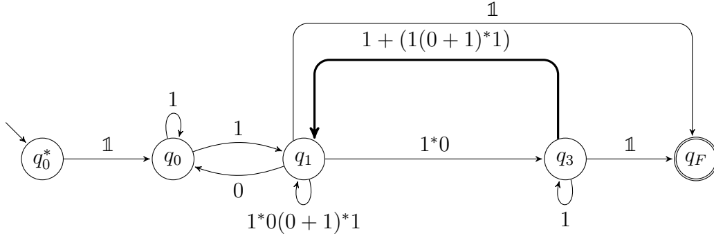
Figure 19: Passo 5, fusione degli archi paralleli da q_3 a q_1 .
