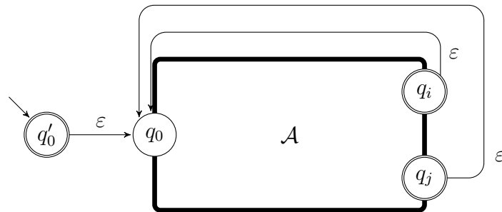
Figure 5: Costruzione dell'automato che decide X^* a partire da quello che decide X .
