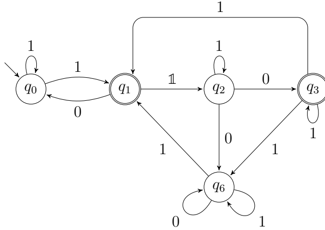
Figure 14: L'automata di partenza visto come automa generalizzato.
