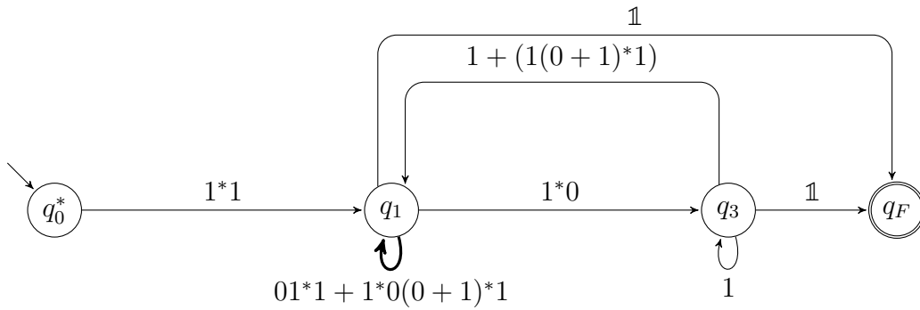
Figure 21: Passo 7, fusione dei due cappi su q_1 .
