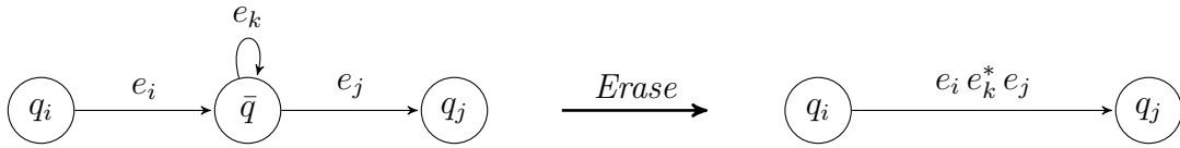
Figure 12: Eliminazione dello stato \bar{q} : il cammino q_i \rightarrow \bar{q} \rightarrow q_j con cappio su \bar{q} diventa un'unica transizione etichettata da e_i e_k^* e_j .
