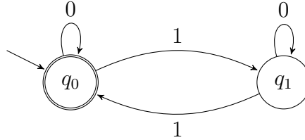
Figure 2: In modo simile all'automa dell'Esempio ?? si può dare l'automa che decide l'insieme di tutte le parole con un numero pari di 1.
