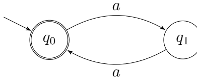
Figure 1: Automa dell'Esempio 2.5, notare che a è un qualsiasi elemento nell'alfabeto A = \{0, 1\} .
