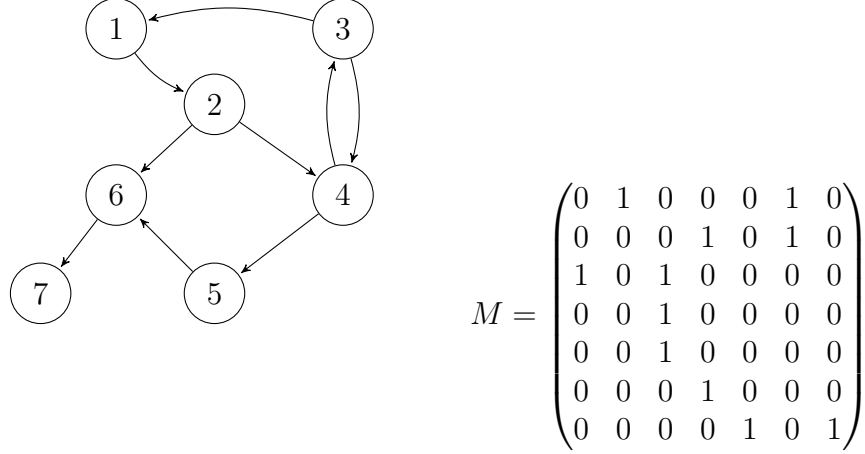
Figure 4: Un generico grafo orientato e la corrispondente matrice di adiacenza.
