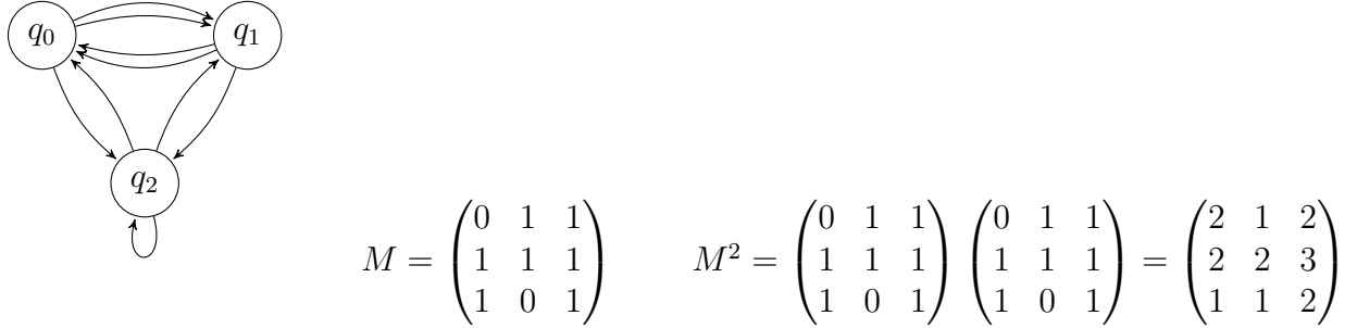
Figure 5: Esempio di grafo orientato (non etichettato). La matrice di adiacenza M e il quadrato M^2 che “conta” il numero di cammini di lunghezza 2 presenti nel grafo.
