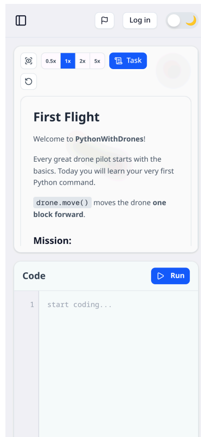
Abb. 7: Die Levelansicht auf einem schmalen Bildschirm. Szene und Editor stehen untereinander statt nebeneinander, der Aufgabentext lässt sich über die Schaltfläche Task ein- und ausblenden.
