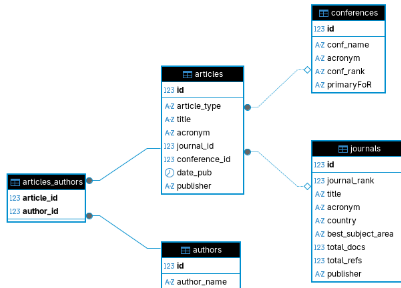
Σχήμα 1.1 Σχεσιακό σχήμα της βάσης δεδομένων του συστήματος
