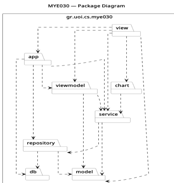
Σχήμα 2.1 Package diagram
