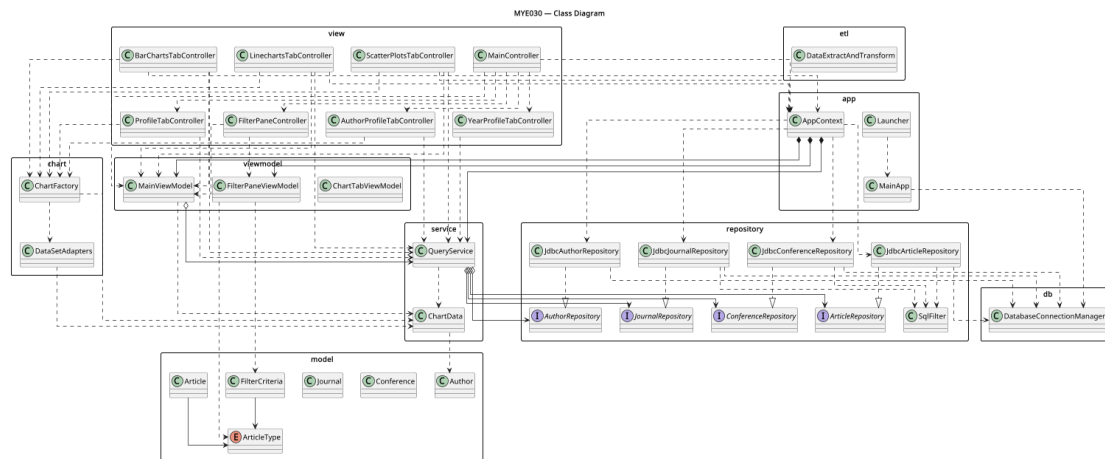
Σχήμα 2.3 Class diagram
