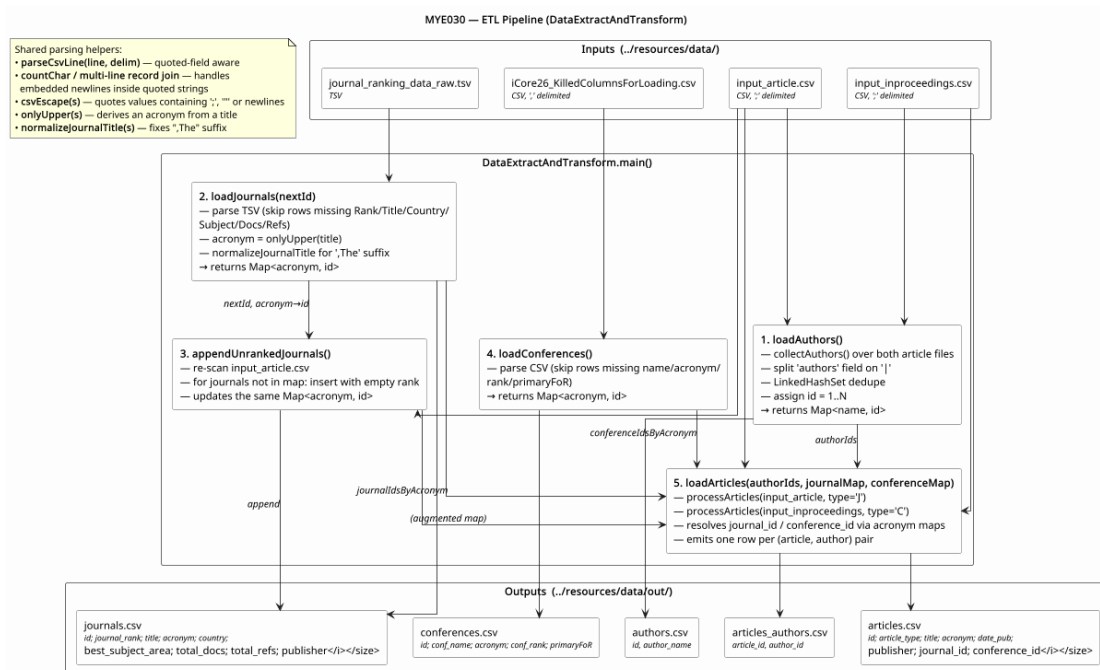
Σχήμα 2. Μετασχηματισμοί ETL με UML diagram
