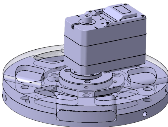
FIGURE 4.5 – Système d'aérofrein d'SP-02 sur CA-TIA
