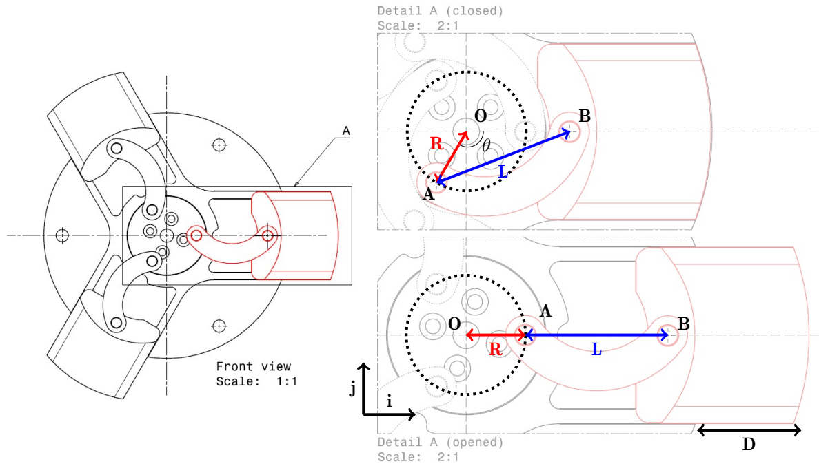
FIGURE 4.8 – Schéma de la cinématique des aérofreins
