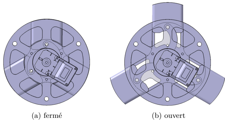
FIGURE 4.6 – Position des aérofreins d'SP-02
