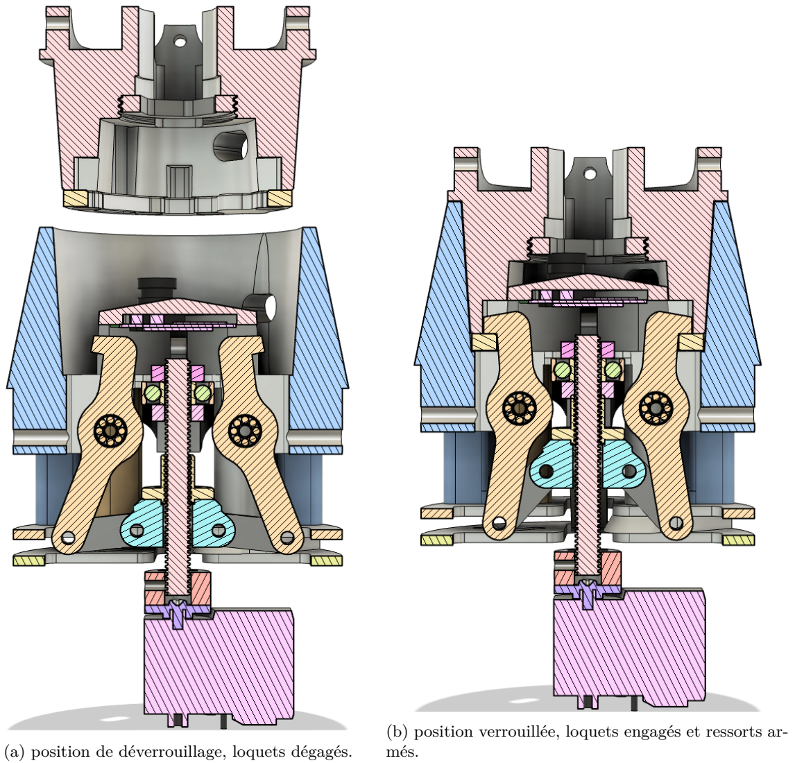
FIGURE 4.10 – Vue en coupe du mécanisme de séparation inter-étages
