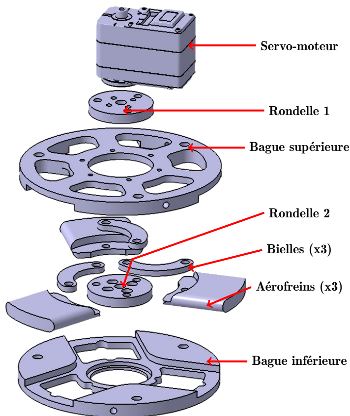
FIGURE 4.7 – Vu éclatée du système d'aérofrein d'SP-02
