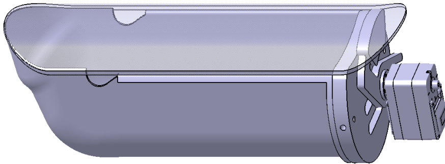
FIGURE 4.9 – Bloc parachute du premier étage sur CATIA
