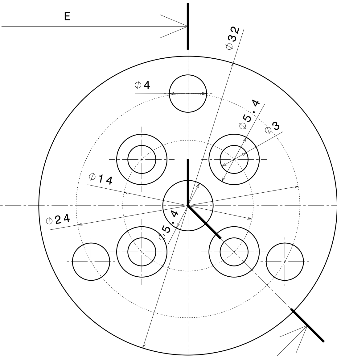
Front view Scale: 4:1
