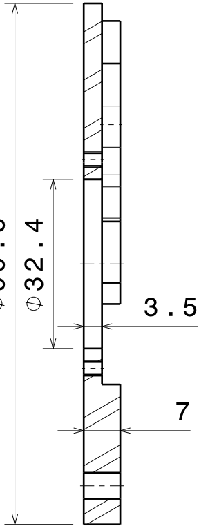
Section view C-C Scale: 1:1
