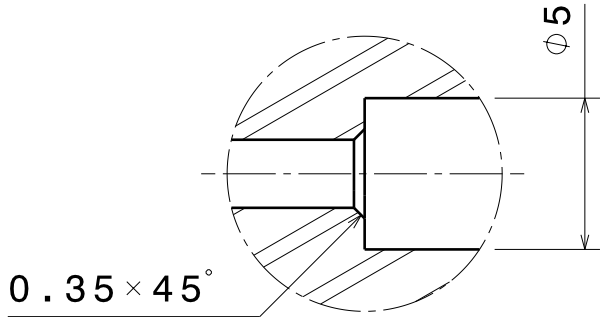
Detail C Scale: 4:1
