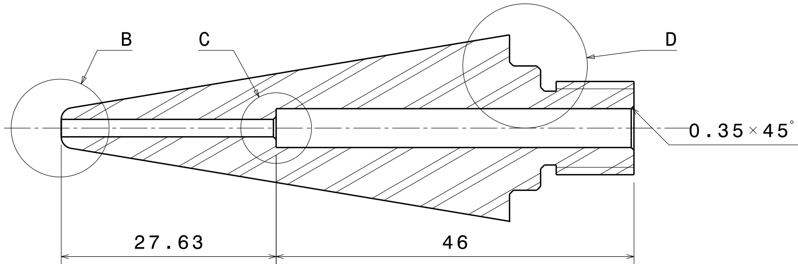
Section view A-A Scale: 2:1
