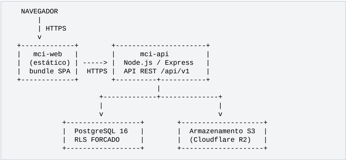
Figura 1 – Topologia de implantação
