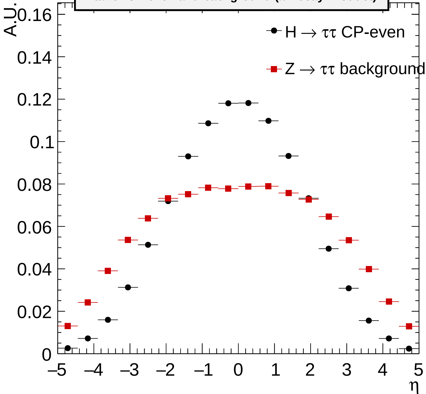
Eta for CP-even and background ( \pi Decay Product)
