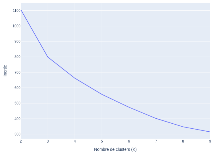
Inertie en fonction du nombre de clusters
