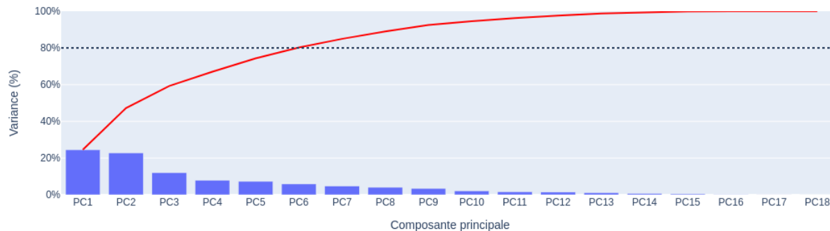
Éboulis des valeurs propres en pourcentage avec cumul et seuil cumulé à 80%
