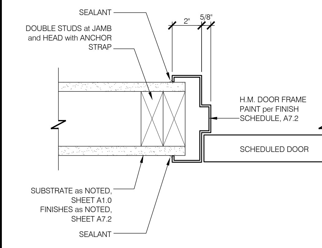
JAMB at INTERIOR. DOOR (HEAD SIM.) 3"=1'-0" 7
