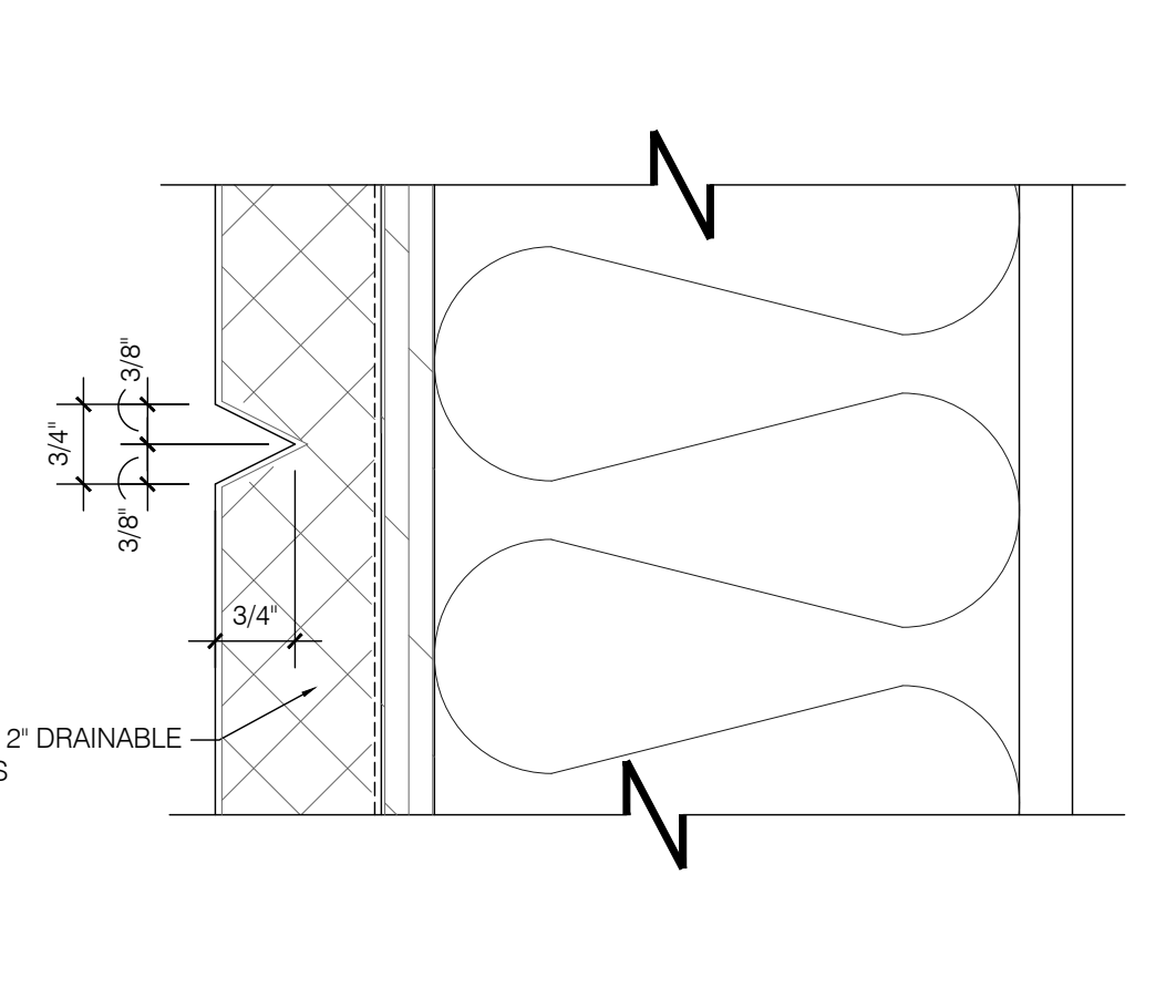
EIFS V-GROOVE 6"-1'-0" 13
