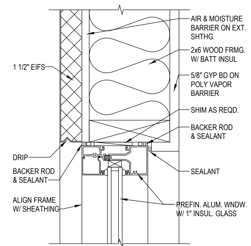
18 WINDOW HEAD DETAIL A-303 SCALE: 3" = 1'-0"
