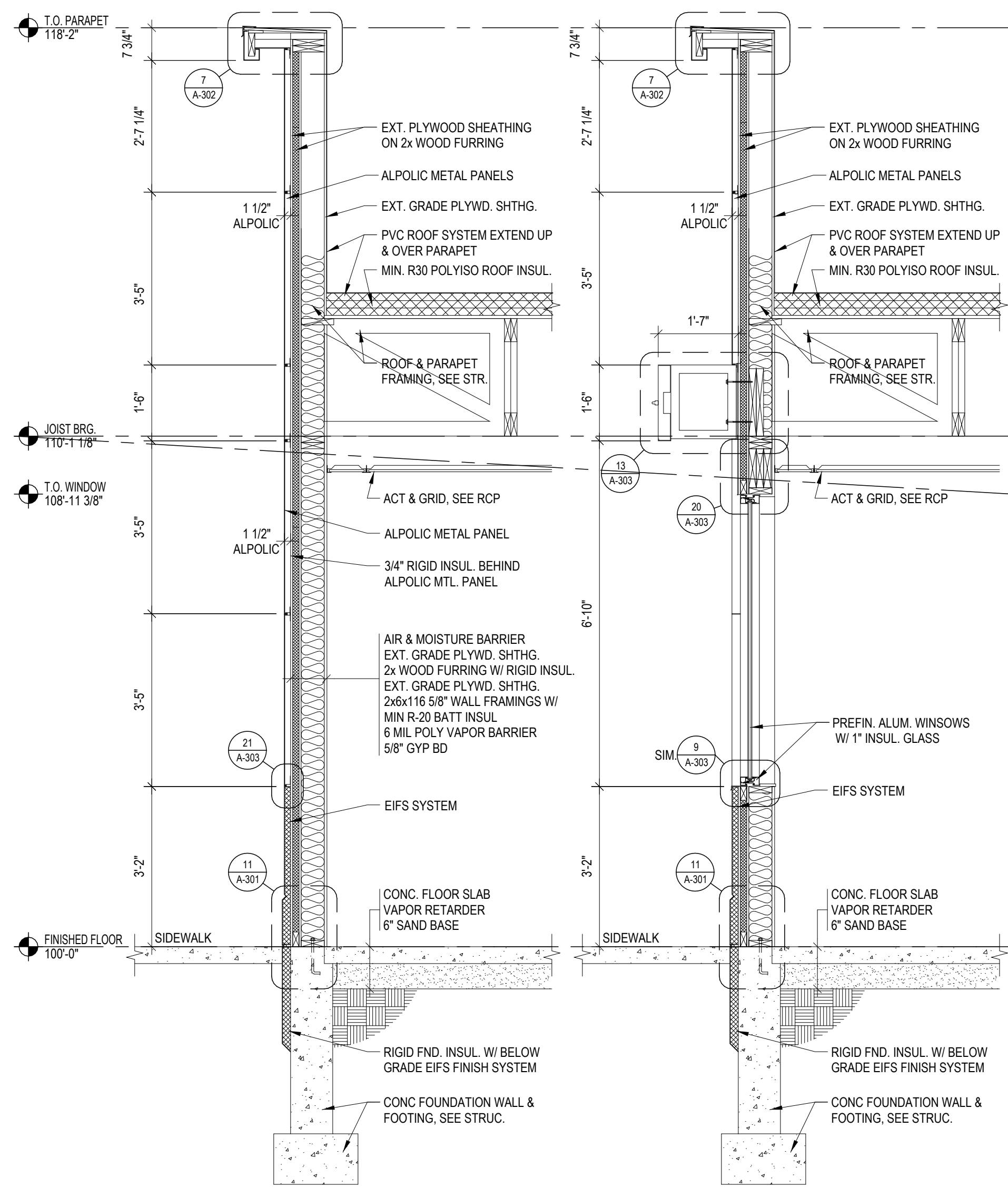
1 SECTION A-303 SCALE: 1/2" = 1'-0"
