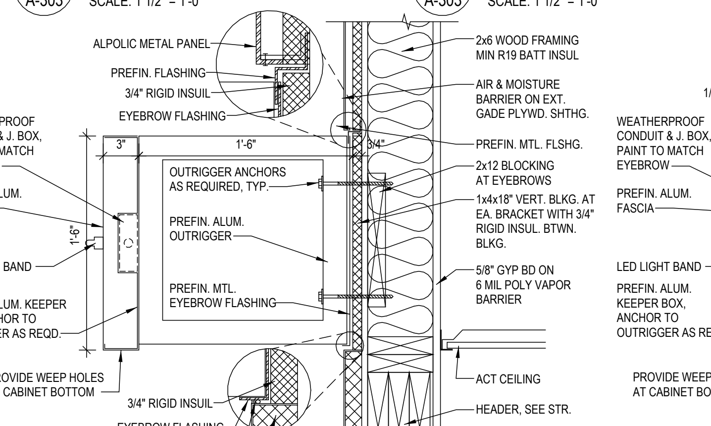
8 DT WINDOW DETAIL A-303 SCALE: 1 1/2" = 1'-0"
