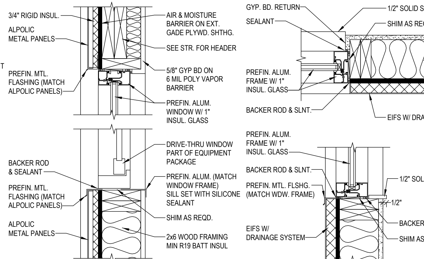
8 DT WINDOW DETAIL A-303 SCALE: 1 1/2" = 1'-0"
