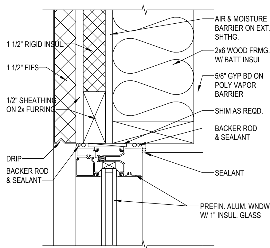
20 WINDOW HEAD DETAIL A-303 SCALE: 3" = 1'-0"
