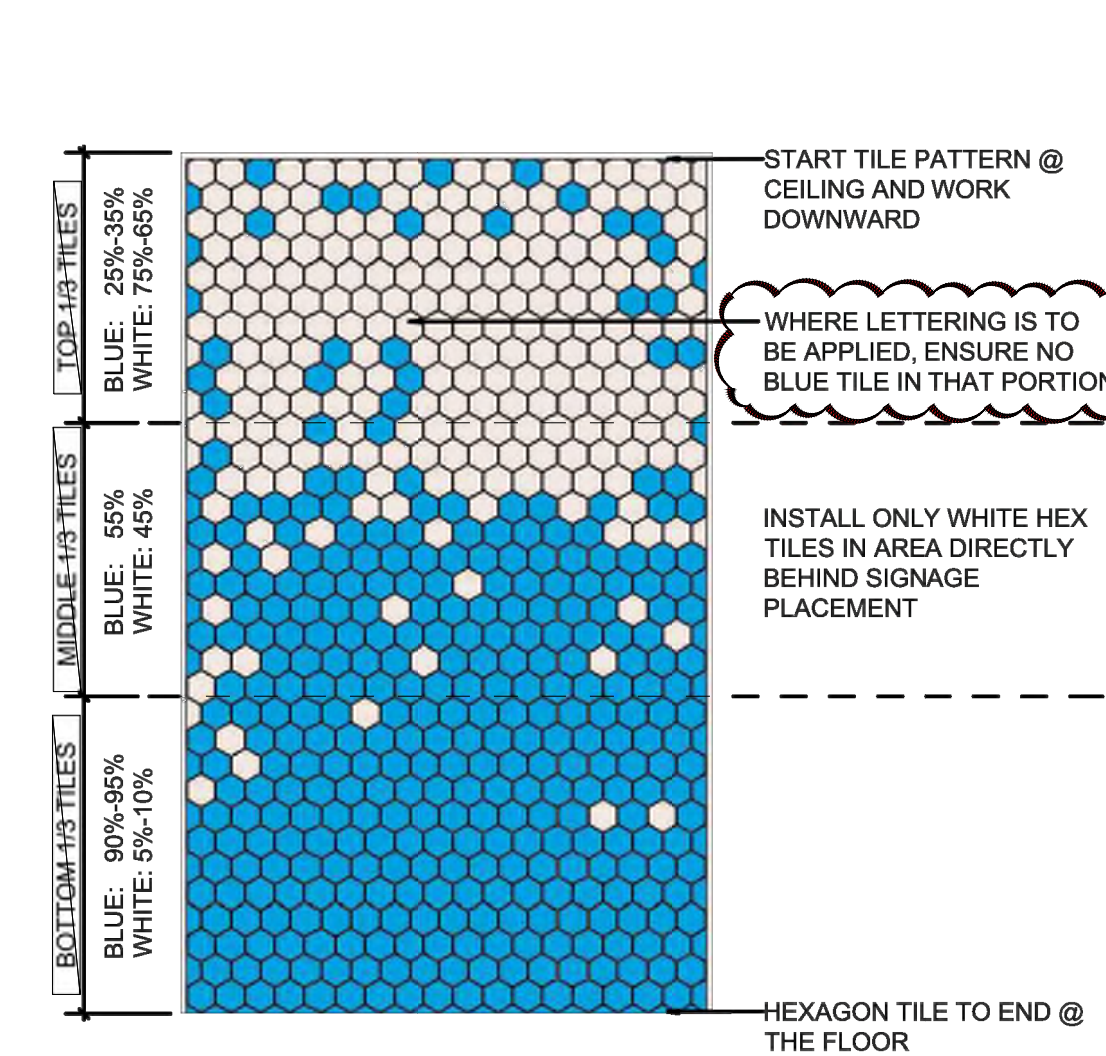
01 HEX TILE LAYOUT SCALE: 1/2" = 1'-0"
