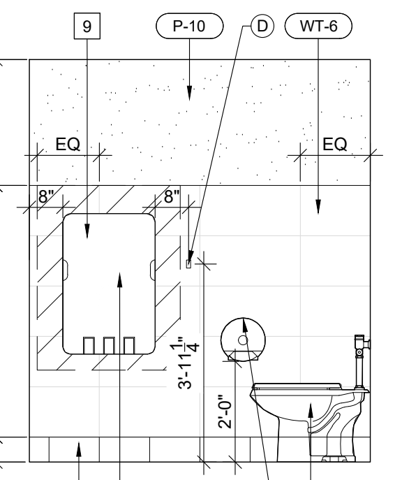
07 UNI-SEX WRM SCALE: 3/8" = 1'-0"
