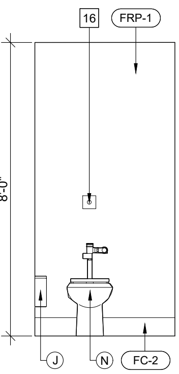
10 STAFF WRM SCALE: 3/8" = 1'-0"
