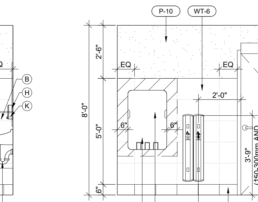
02 UNIVERSAL UNI-SEX WRM SCALE: 3/8" = 1'-0"
