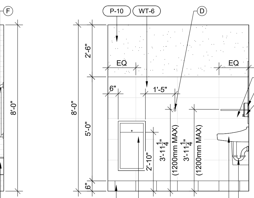
03 UNIVERSAL UNI-SEX WRM SCALE: 3/8" = 1'-0"
