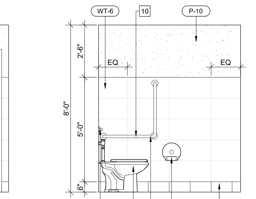
01 UNIVERSAL UNI-SEX WRM SCALE: 3/8" = 1'-0"
