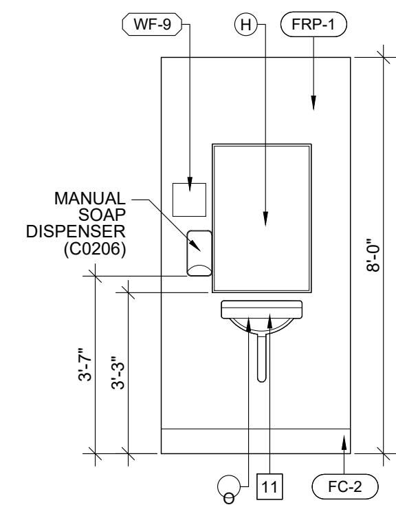
12 STAFF WRM SCALE: 3/8" = 1'-0"
