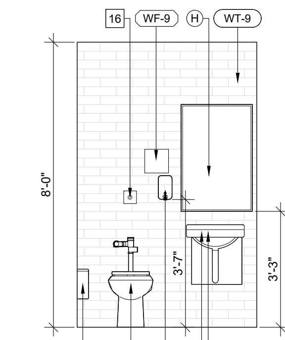
08 UNI-SEX WRM SCALE: 3/8" = 1'-0"
