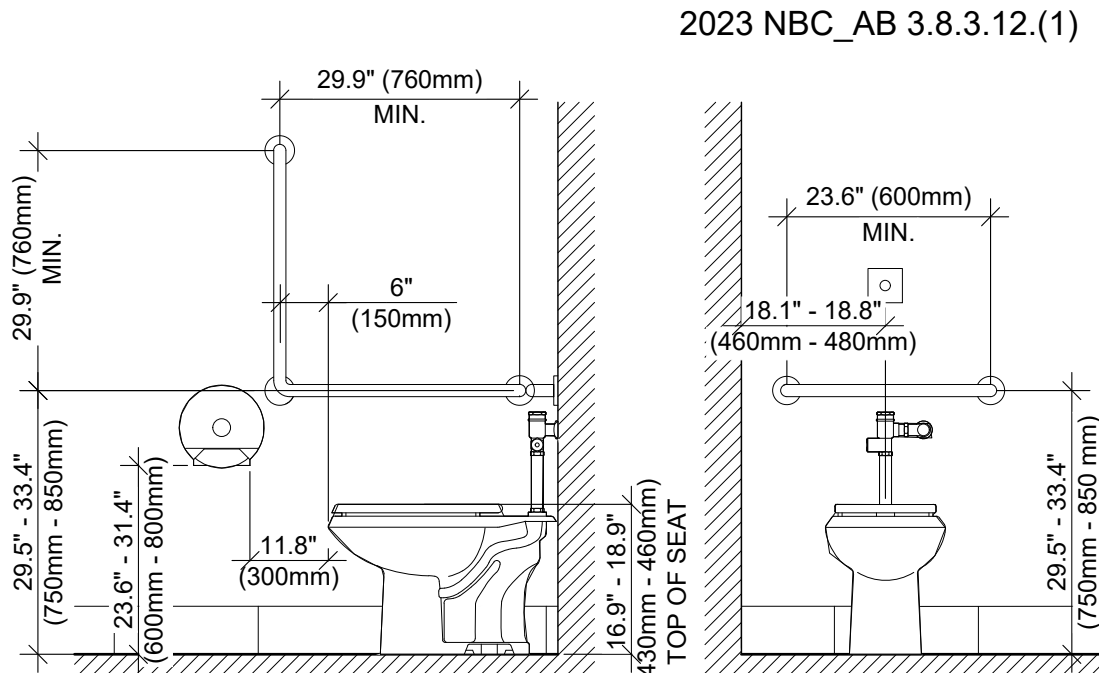
13 GRAB BAR DETL SCALE: 1/2" = 1'-0"
