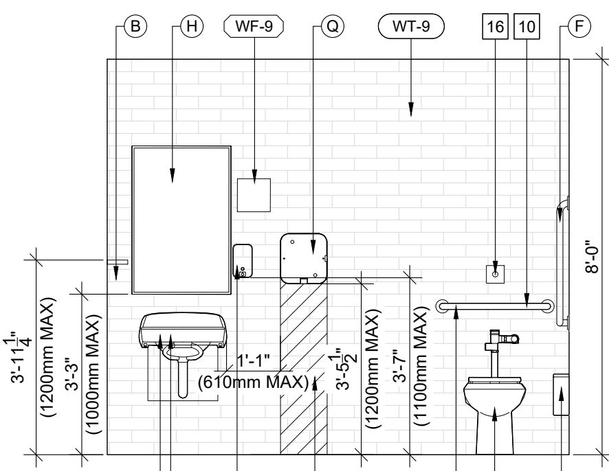
04 UNIVERSAL UNI-SEX WRM SCALE: 3/8" = 1'-0"
