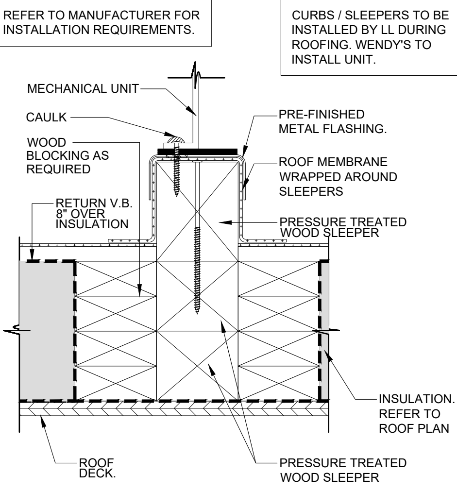
04 CONDENSER UNIT DETAIL SCALE: 3" = 1'-0"
