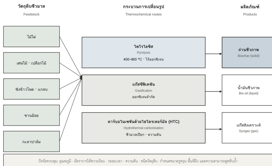
ภาพที่ 1-2 เส้นทางการผลิตถ่านชีวภาพจากชีวมวลด้วยไพโรไลซิส แก๊สซิฟิเคชัน และคาร์บอไนเซชันด้วยไฮโดรเทอร์มัล (ผู้วิจัยวาดใหม่ตาม [7])
