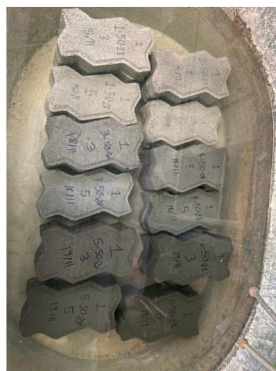
ข) การทดสอบการดูดซึมน้ำ (72-hour Water Absorption (%))
