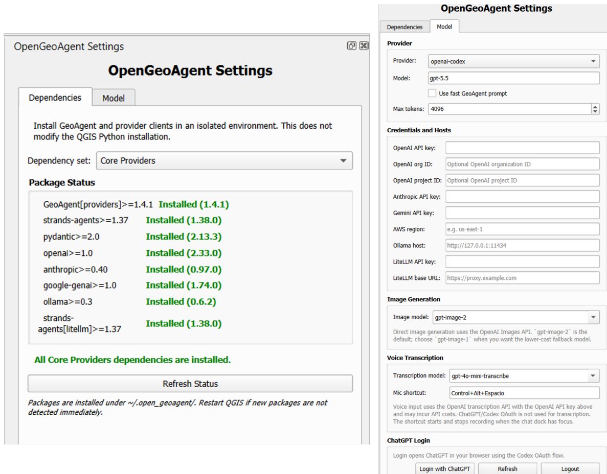
Figura 1: Pantallazo del Panel de Configuración de OpenGeoAgent
