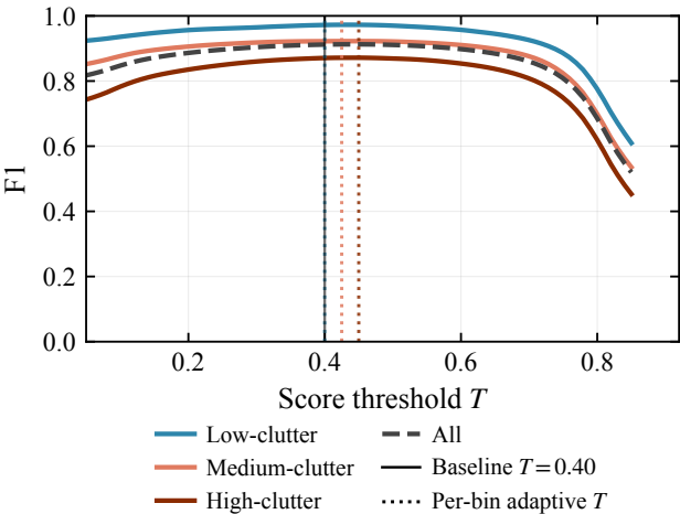
SARDet-100K: F1
