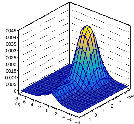
D^+D^- OS - SS, 0-20%, per trigger
