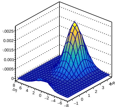
B^+B^- OS - SS, 0-20%, per trigger
