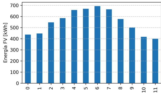
Figura 7: (G3) Producción de energía mensual.
