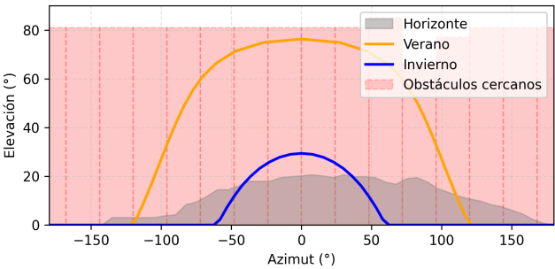
Figura 2: (G1) Perfil del horizonte y sombras.
