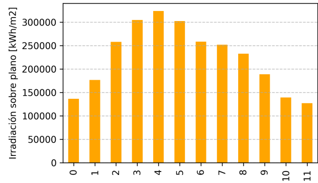
Figura 4: (G1) Irradiación mensual sobre plano fijo.
