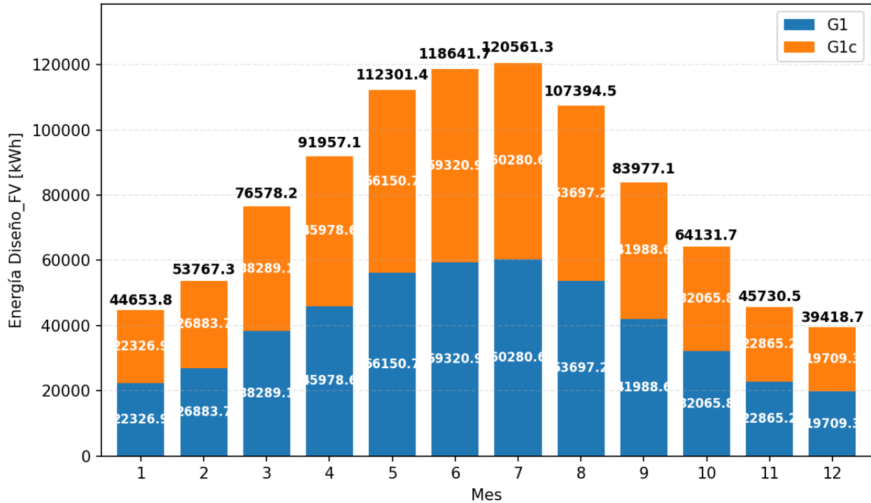
Producción de energía mensual del sistema Diseño_FV
