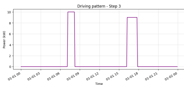
Figura 7: Driving Pattern - Conectar el vehículo eléctrico como carga P3
