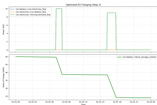
Figura 9: Results - Conectar el vehículo eléctrico como carga P3
