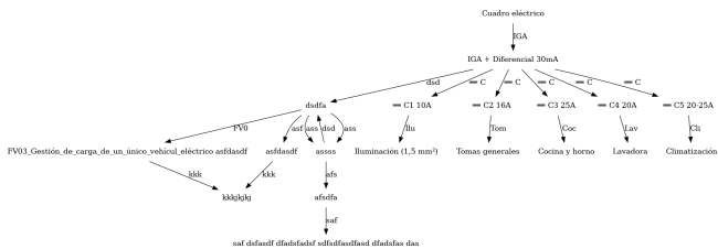
Figura 16: esquema electrico
