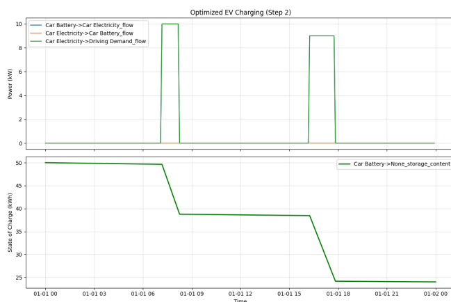
Figura 6: Results - Conectar el vehículo eléctrico como carga P2
