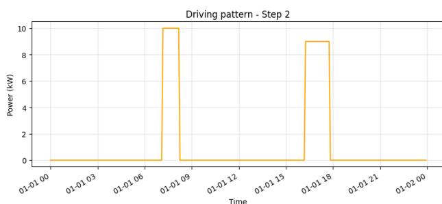
Figura 4: Driving Pattern - Conectar el vehículo eléctrico como carga P2
