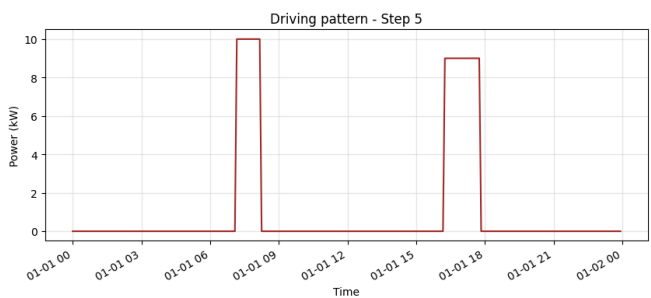
Figura 13: Driving Pattern - Conectar el vehículo eléctrico como carga P5
