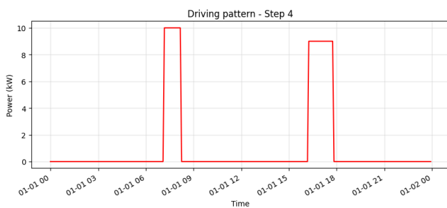
Figura 10: Driving Pattern - Conectar el vehículo eléctrico como carga P4
