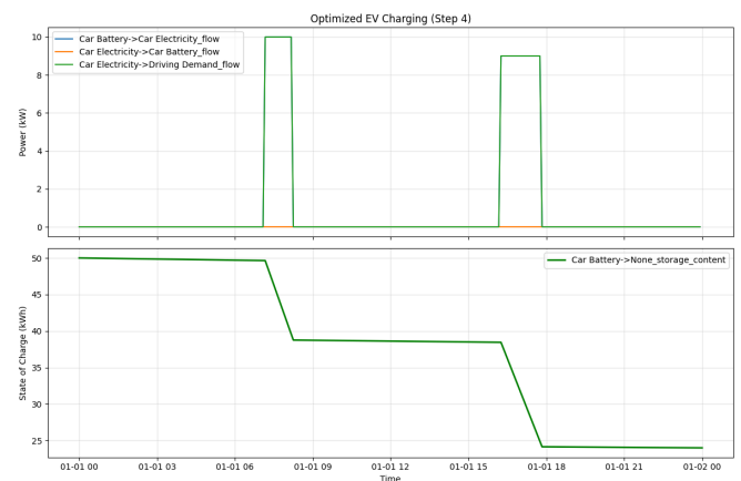
Figura 12: Results - Conectar el vehículo eléctrico como carga P4
