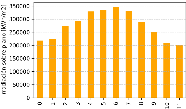
Figura 4: (G3) Irradiación mensual sobre plano fijo.
