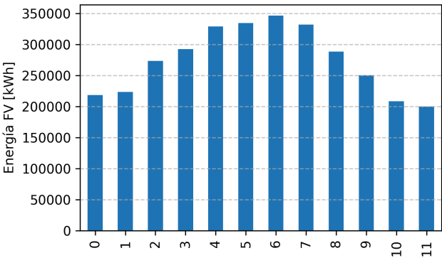
Figura 3: (G3) Producción de energía mensual.
