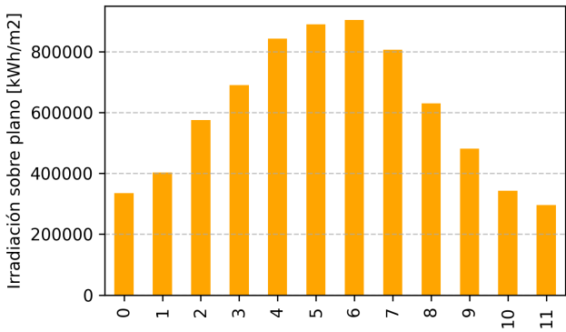
Figura 8: (G2) Irradiación mensual sobre plano fijo.
