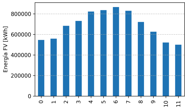
Figura 11: (G3) Producción de energía mensual.
