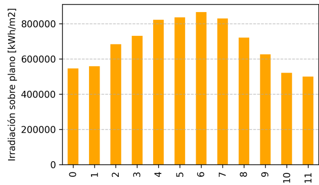
Figura 12: (G3) Irradiación mensual sobre plano fijo.
