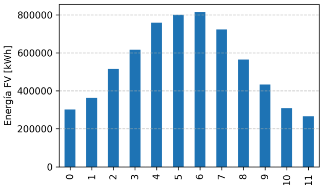
Figura 3: (G1) Producción de energía mensual.
