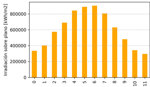
Figura 8: (G2) Irradiación mensual sobre plano fijo.
