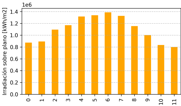
Figura 12: (G3) Irradiación mensual sobre plano fijo.
