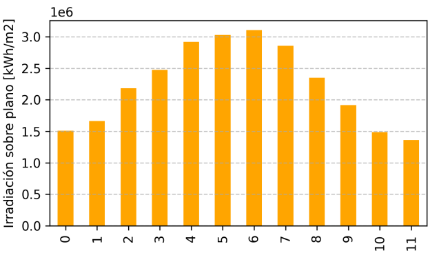
Figura 15: (Total) Irradiación mensual sobre plano fijo.
