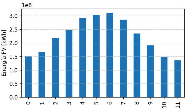
Figura 14: (Total) Producción de energía mensual.
