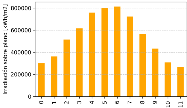
Figura 4: (G1) Irradiación mensual sobre plano fijo.
