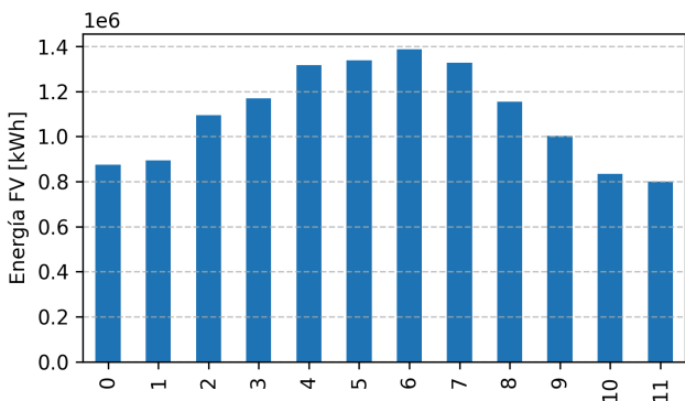
Figura 11: (G3) Producción de energía mensual.
