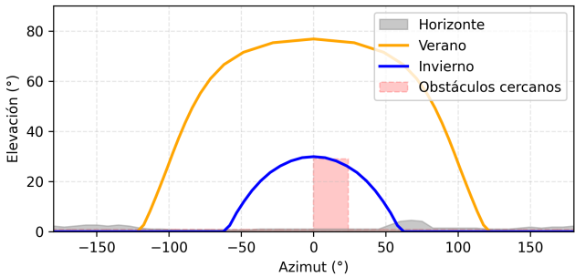
Figura 6: (G2) Perfil del horizonte y sombras.
