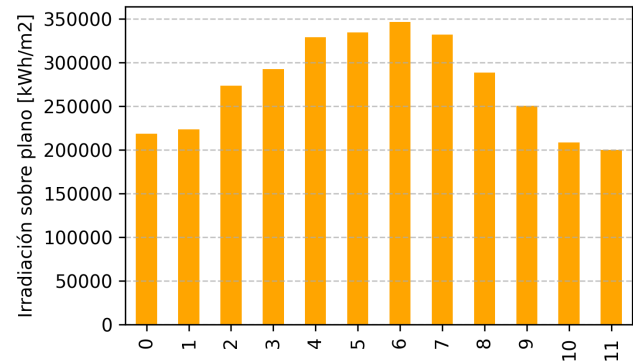
Figura 7: (Total) Irradiación mensual sobre plano fijo.
