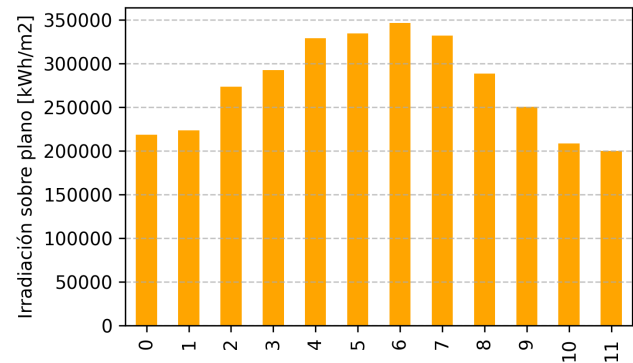
Figura 4: (G3) Irradiación mensual sobre plano fijo.
