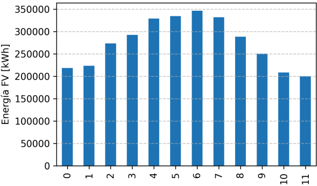
Figura 6: (Total) Producción de energía mensual.
