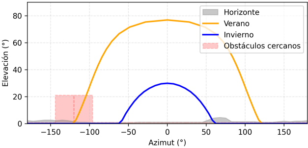
Figura 2: (G3) Perfil del horizonte y sombras.
