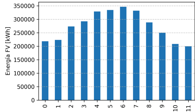
Figura 3: (G3) Producción de energía mensual.
