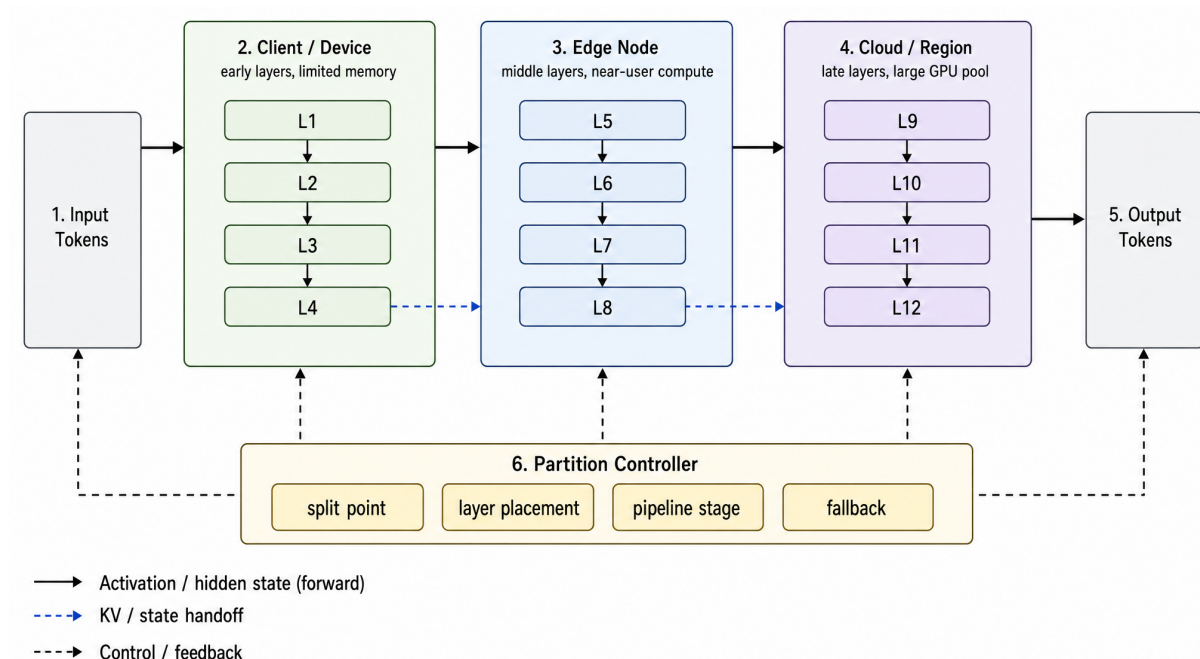
图 7 Layer-wise / Vertical Partitioning 机制示意图
