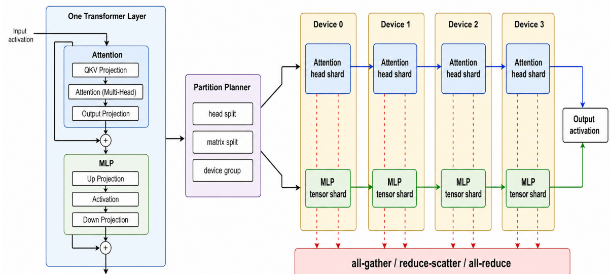
图 8 Tensor / Operator-level Partitioning 机制示意图
