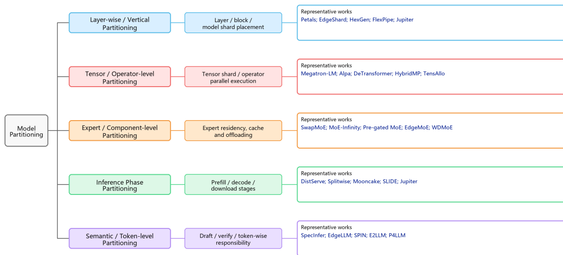
图6 CEC 下资源自适应模型切分部署方法的分类树
