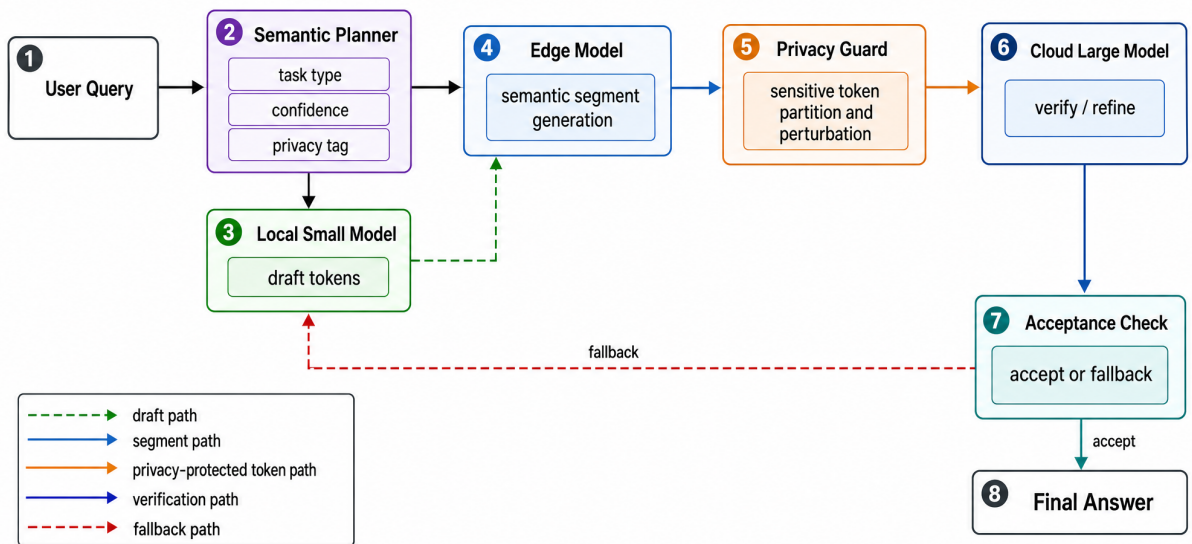
图 11 Semantic / Token-level Partitioning 机制示意图
