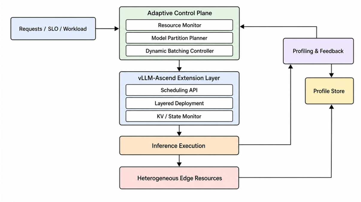
图 17 基于 vLLM-Ascend 的资源自适应模型切分部署工程框架
