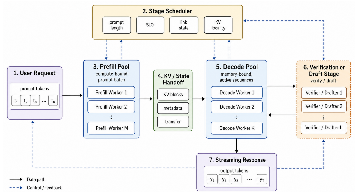
图 10 Inference Phase Partitioning 机制示意图
