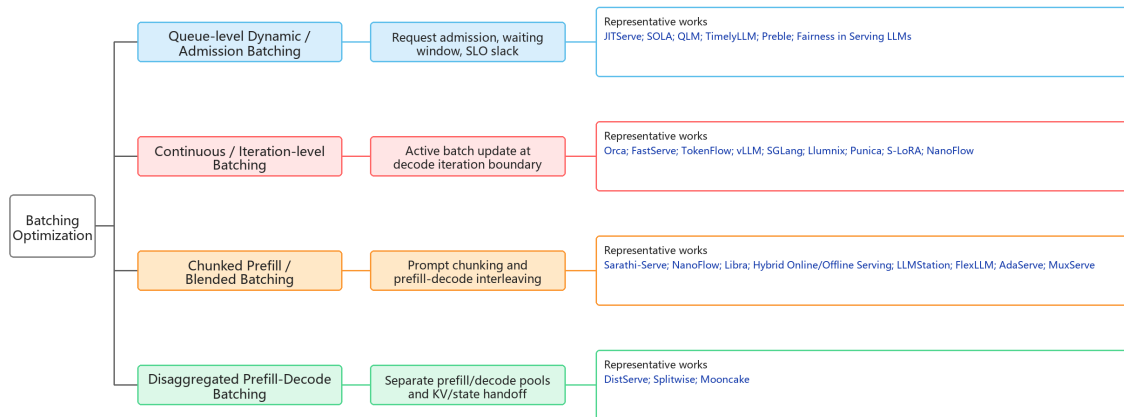
图 12 CEC 下业务感知 Batching 参数优化方法的分类树
