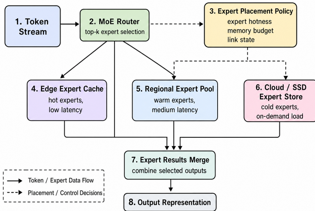
图 9 Expert / Component-level Partitioning 机制示意图
