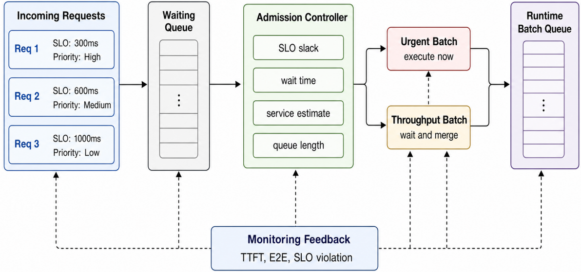
图 13 Queue-level Dynamic / Admission Batching 机制示意图
