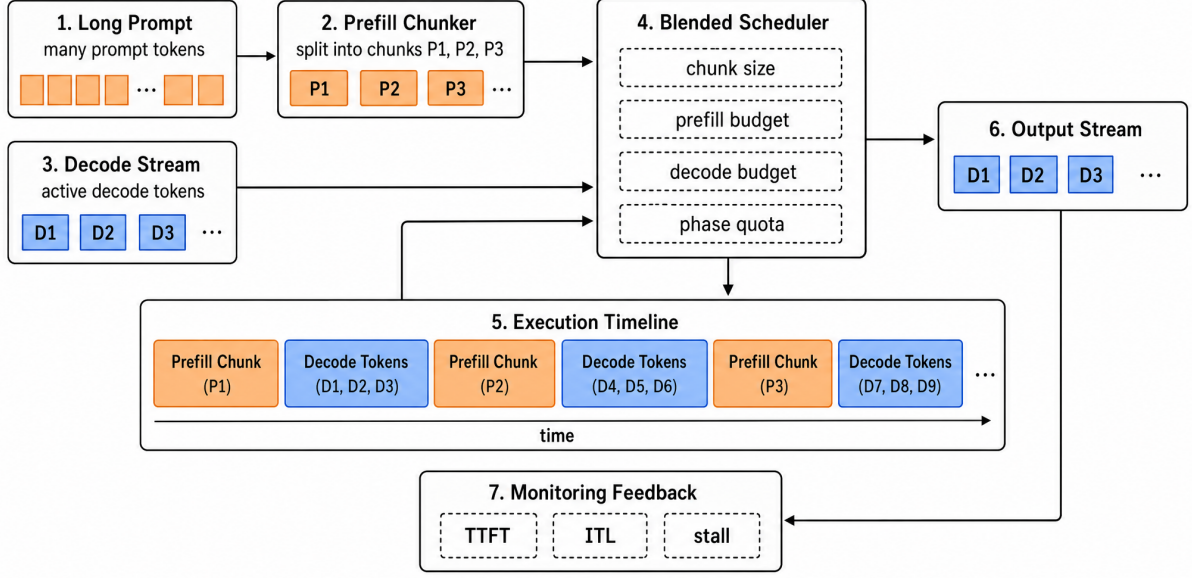
图 15 Chunked Prefill / Blended Batching 机制示意图
