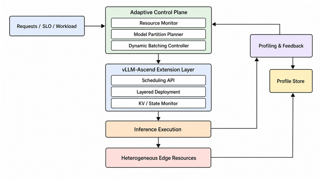
图 22 面向 Ascend/CANN 验证环境的 CEC 推理工程框架
