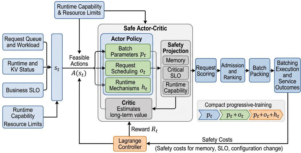
图 20 基于拉格朗日约束和安全投影的在线 batching 优化架构
