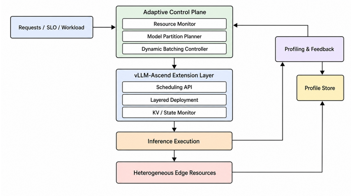
图 18 基于 vLLM-Ascend 的资源自适应模型切分部署工程框架
