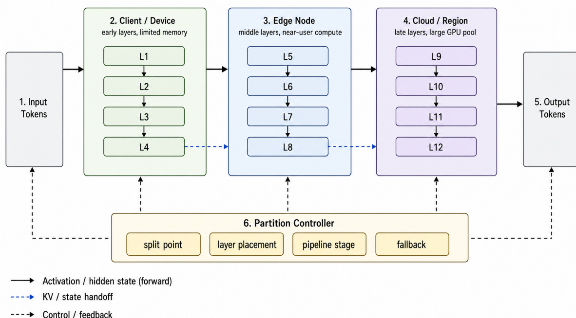
图 7 Layer-wise / Vertical Partitioning 机制示意图
