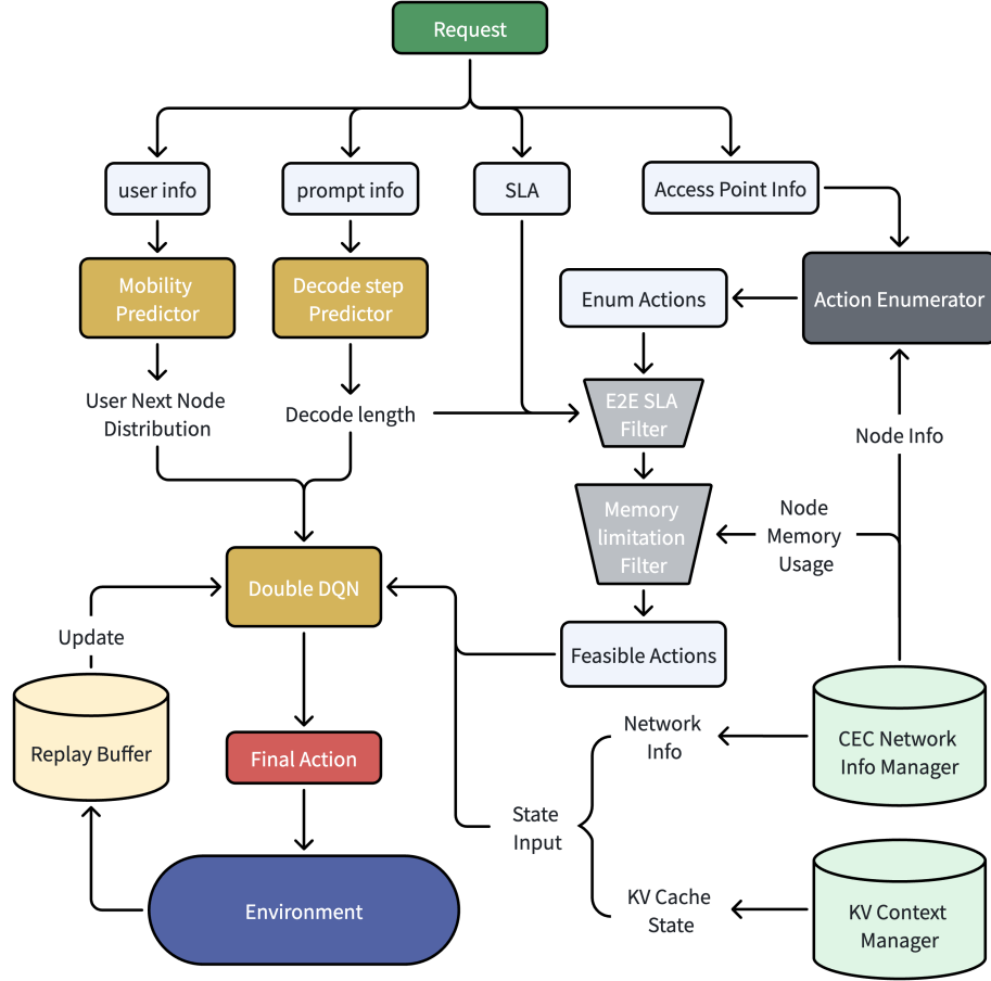
图 17 单个请求到达后的长期成本感知卸载决策流程。Request 被拆分为用户信息、prompt 信息和 SLA 信息：用户信息进入 mobility predictor 得到未来入口分布，prompt 信息进入 output length predictor 得到 decode 长度估计，SLA 作为动作过滤约束。CEC system state 与 KV context manager 提供节点负载、链路带宽、显存和 KV block 位置/版本等状态。State builder 将上述信息组合为决策输入；action enumerator 枚举“计算节点 + KV 获取方式”候选，per-action estimator 逐动作估计通信、KV 同步/重算、prefill、decode 和显存开销。E2E SLA filter 与 Memory/KV filter 先剔除不可行动作，Double DQN router 再在 feasible actions 中比较长期成本并输出 final action。环境执行后的实际时延、输出长度、KV 增量和显存变化写入 replay buffer，用于更新预测器、估计器和路由策略。
