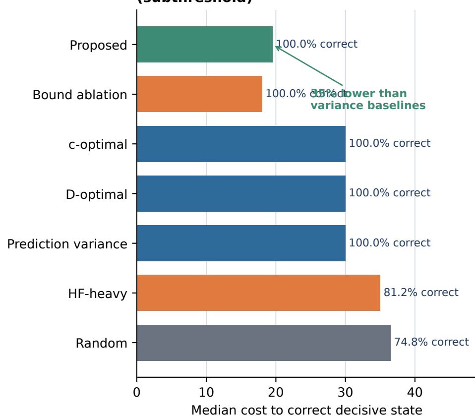
(b) True contrast \Delta = 2 (subthreshold)
