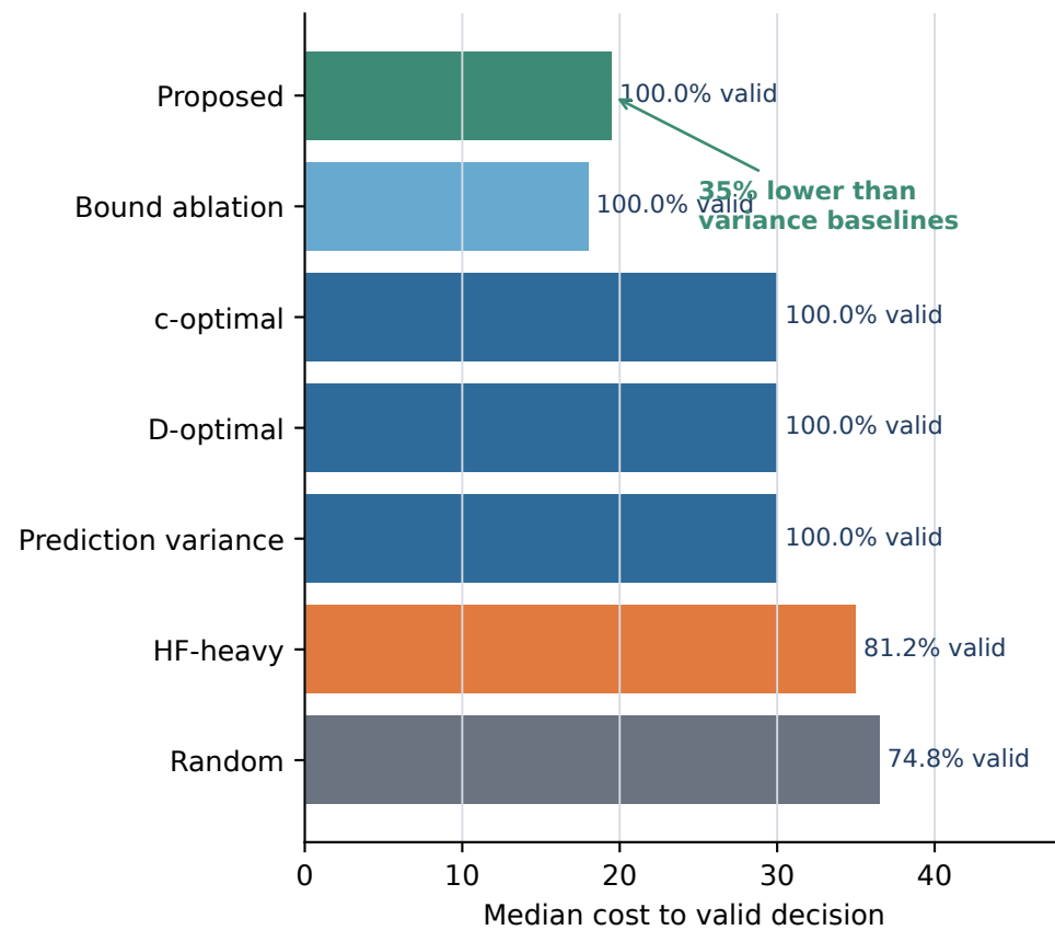
(b) True contrast \Delta=2
