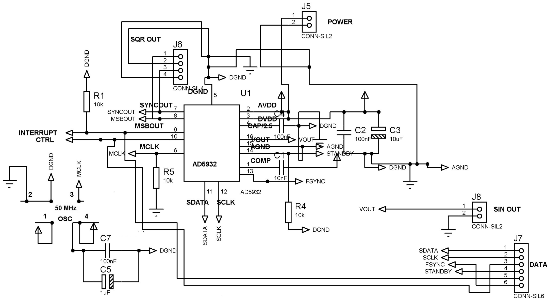
DDS MODULE
