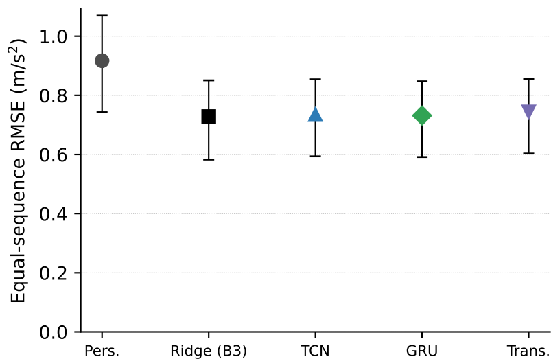
EuRoC → UZH (n=8)
