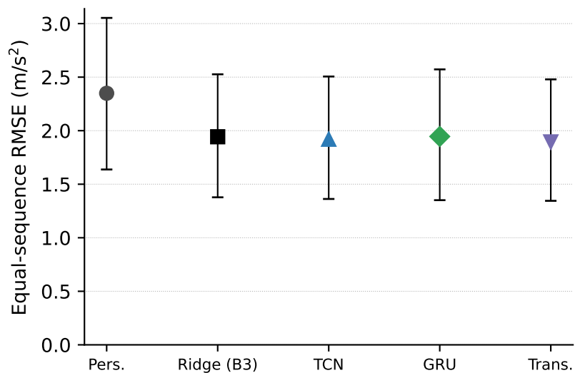
UZH → EuRoC (n=6)
