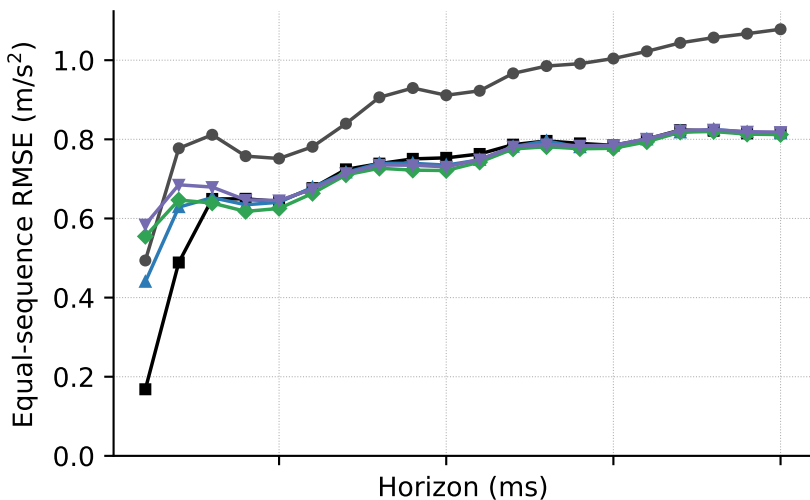
EuRoC \rightarrow UZH (n=8)
