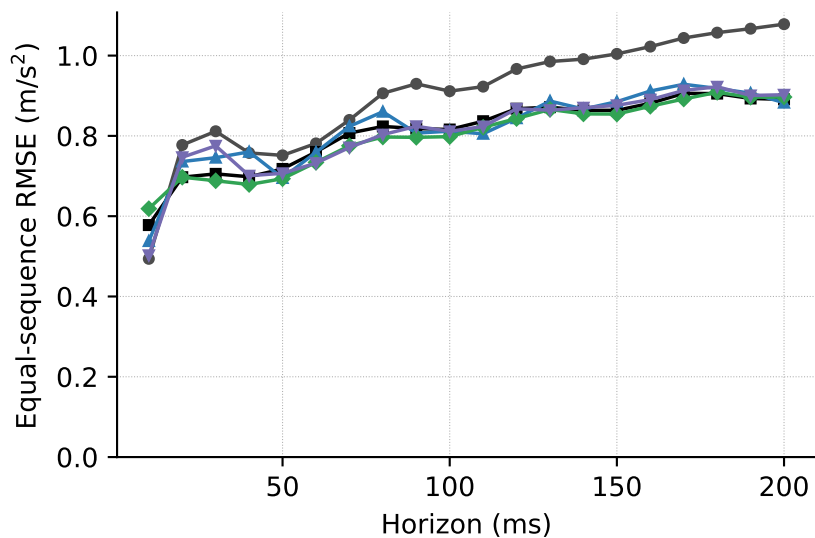
UZH \rightarrow EuRoC (n=6)
