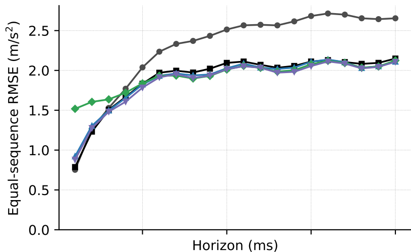
UZH \rightarrow EuRoC (n=6)
