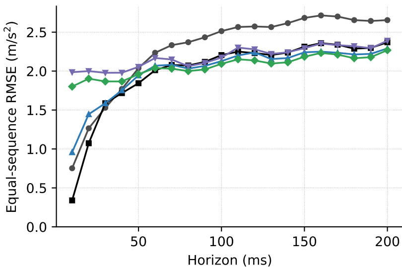
EuRoC \rightarrow UZH (n=8)
