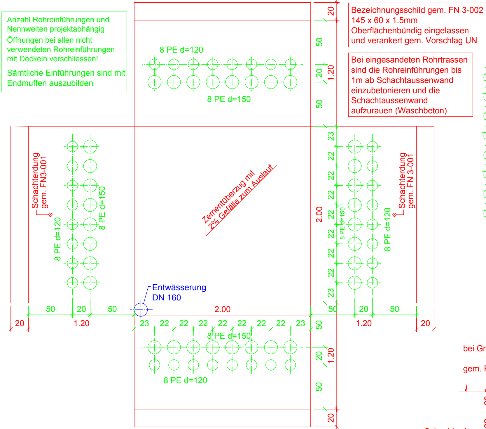
Abwicklung 1:25
