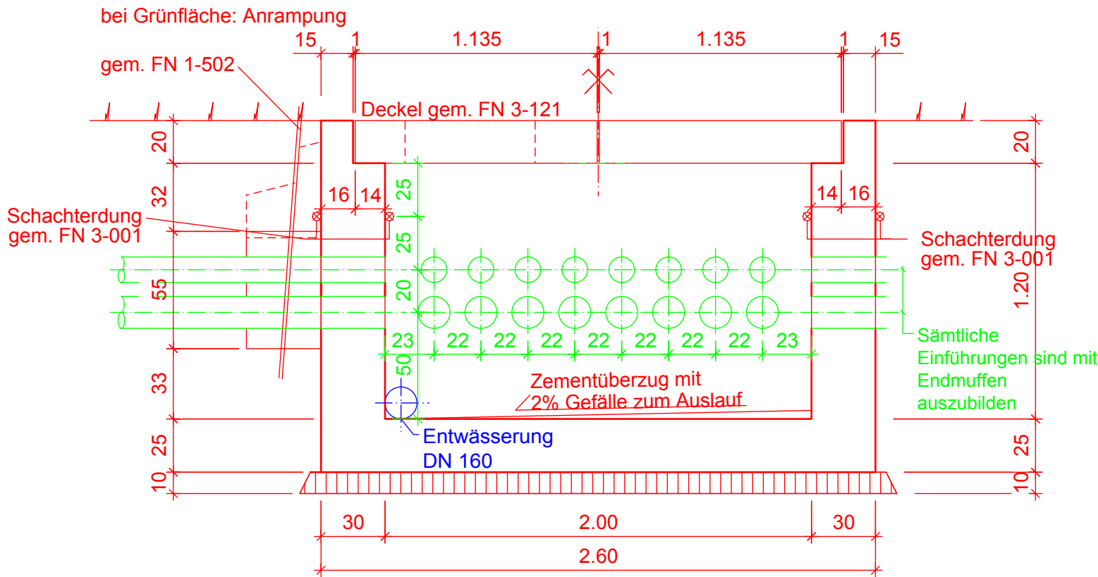
Querschnitt 1:25
