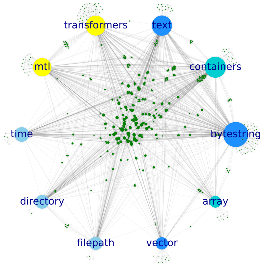
LTS 0-7
