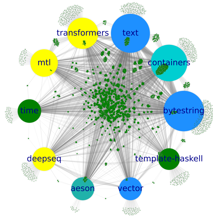
LTS 24-11
