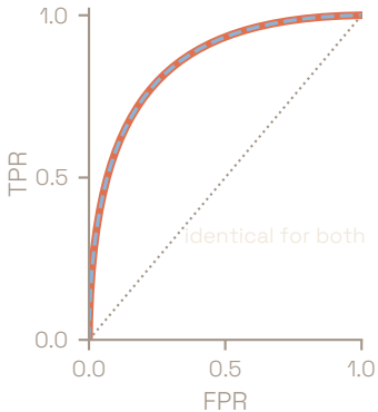
ROC
